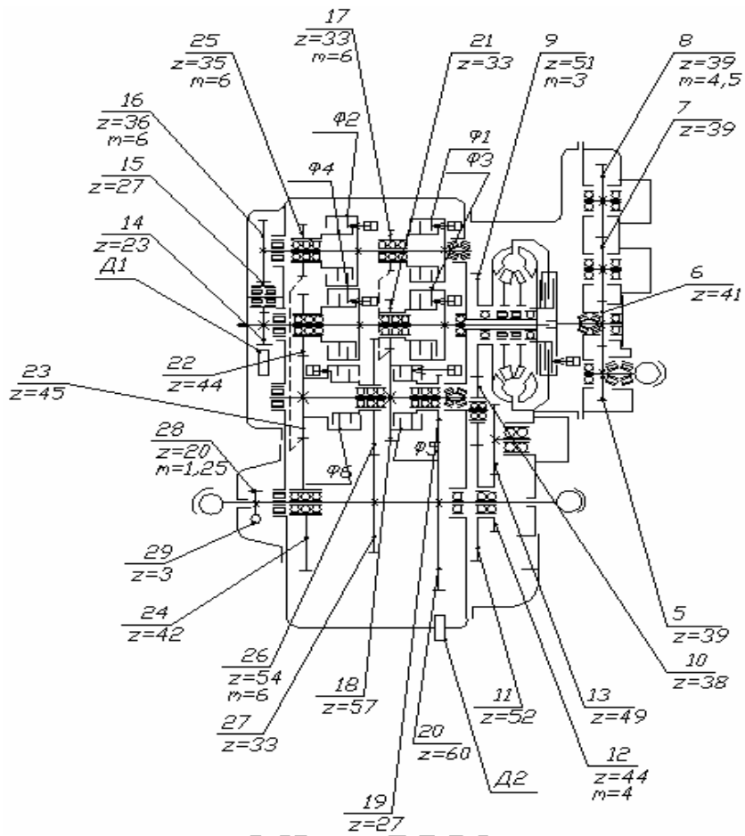
Рис. 1. Схема установки датчиков на ГМКП МоА3-4048
