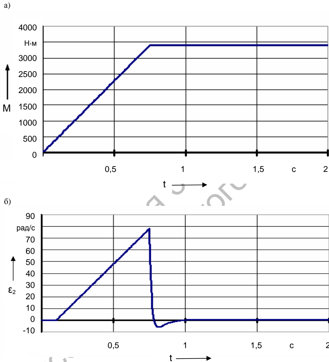
Рис. 5. Результаты моделирования процесса включения фрикциона: а – изменение момента трения фрикциона при замыкании M_f ; б – изменение углового ускорения выходного вала \epsilon_2
