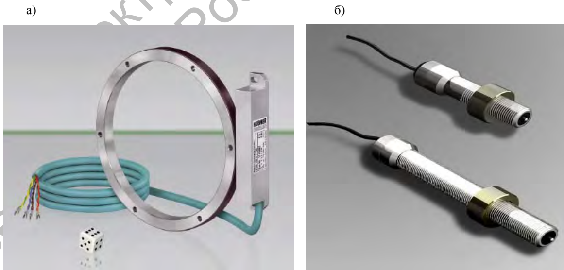
Рис. 2. Датчики системы диагностики гидромеханической трансмиссии МоА3-4048: а – магнитный инкрементальный энкодер МНГ 150; б – импульсные датчики скорости фирмы «Хоневел» серии 3015
