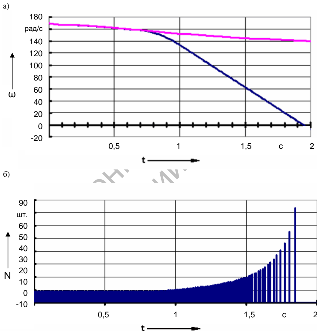
Рис. 6. Результаты моделирования процесса буксования фрикциона: а – изменения угловой скорости ведущей и ведомой частей фрикциона при буксовании; б – изменение числа импульсов опорного сигнала за поворот выходной шестерни на один зуб
