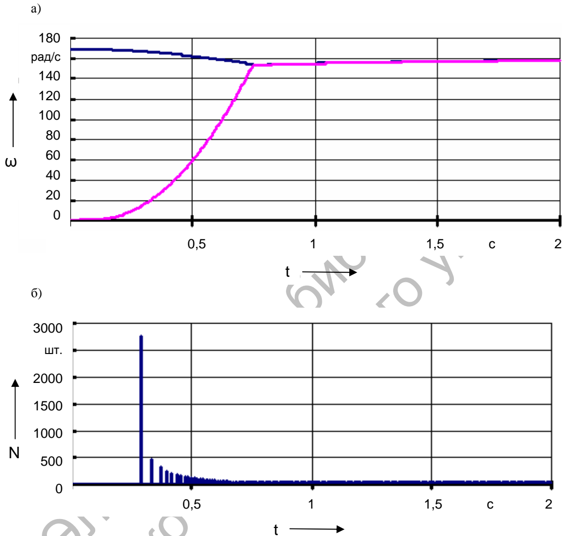
Рис. 4. Результаты моделирования процесса включения фрикциона: а – изменение угловых скоростей ведущей и ведомой частей фрикциона при замыкании; б – изменение числа импульсов опорного сигнала за поворот выходной шестерни на один зуб при замыкании фрикциона
