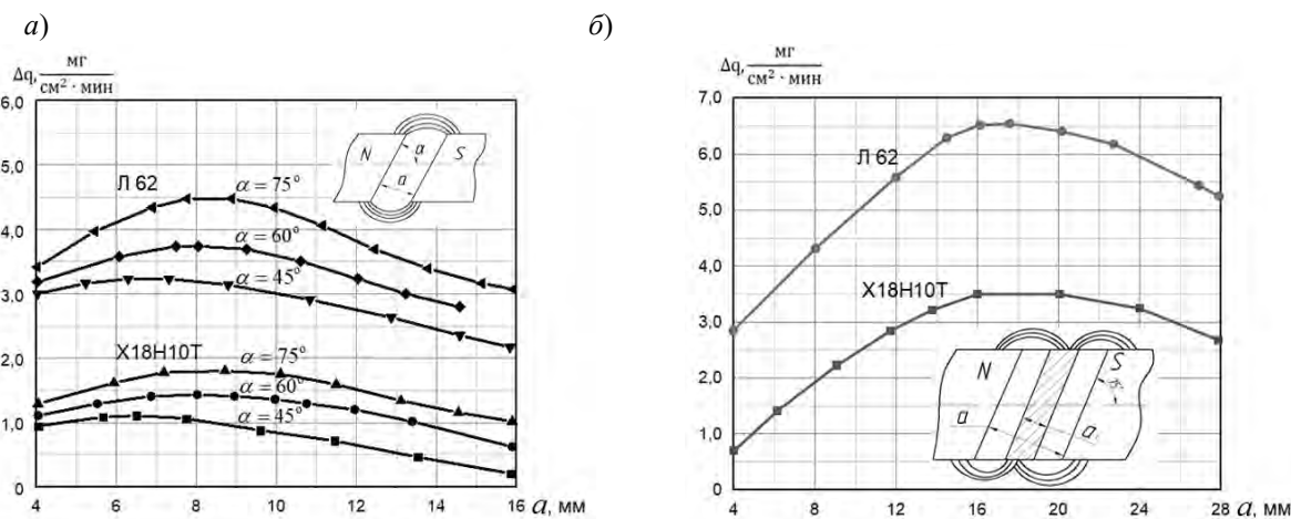
Рис. 2. Зависимость удельного сьема материала ( \Delta q ) при обработке индуктором с обычным (а) и увеличенным (б) межполюсным зазором ( \alpha = 75^\circ )
