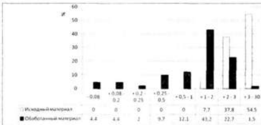
Рис. 2. Результаты измельчения цементного клинкера
