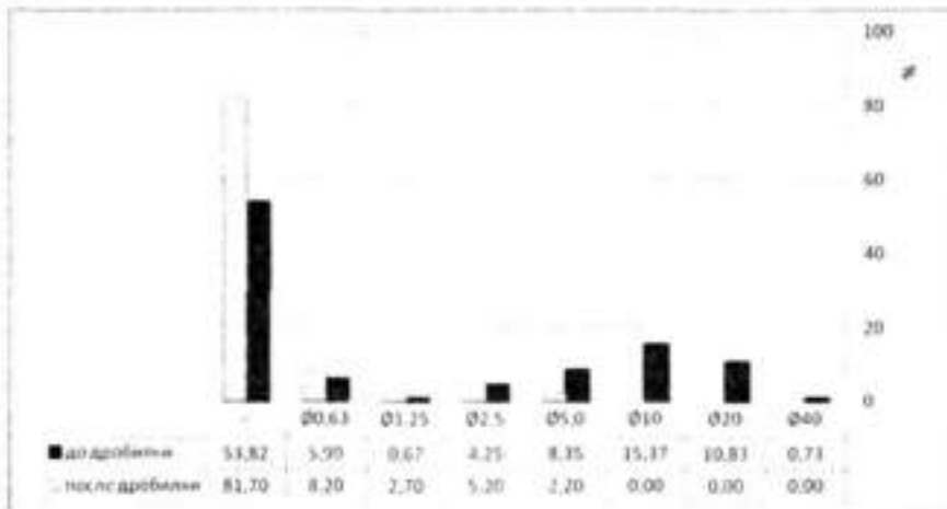
Рис. 1. Результаты измельчения отходов газосиликатных изделий
