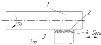
Рис. 1. Схема магнитно-абразивной обработки с наложением ультразвуковых колебаний: 1 – обрабатываемая деталь; 2 – ферромагнитный порошок; 3 – полюсный наконечник; 4 – пружинная пластина
