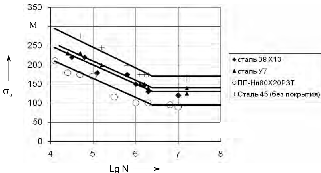
Рис. 4. Кривые усталости образцов с наплавленными покрытиями: 1 – сталь 08X13 (♦); 2 – сталь У7 (▲); 3 – ПП-Нп-80X20P3Т (○)
