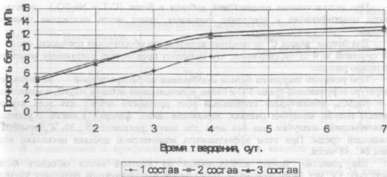
Рис. 1. График роста прочности бетона в течении 7 суток
