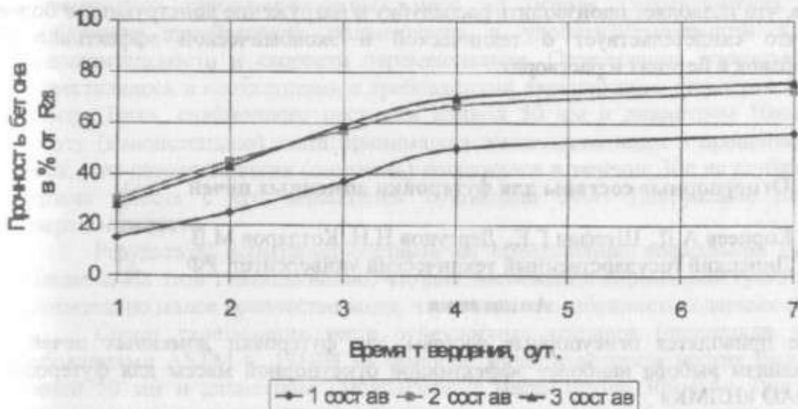
Рис. 3. Кинетика роста прочности бетона
