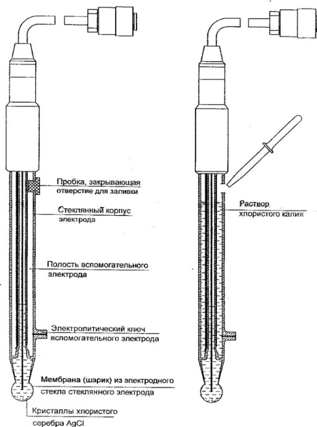
Рисунок 3.2 – Комбинированный электрод ЭСКЛ.08М.1
