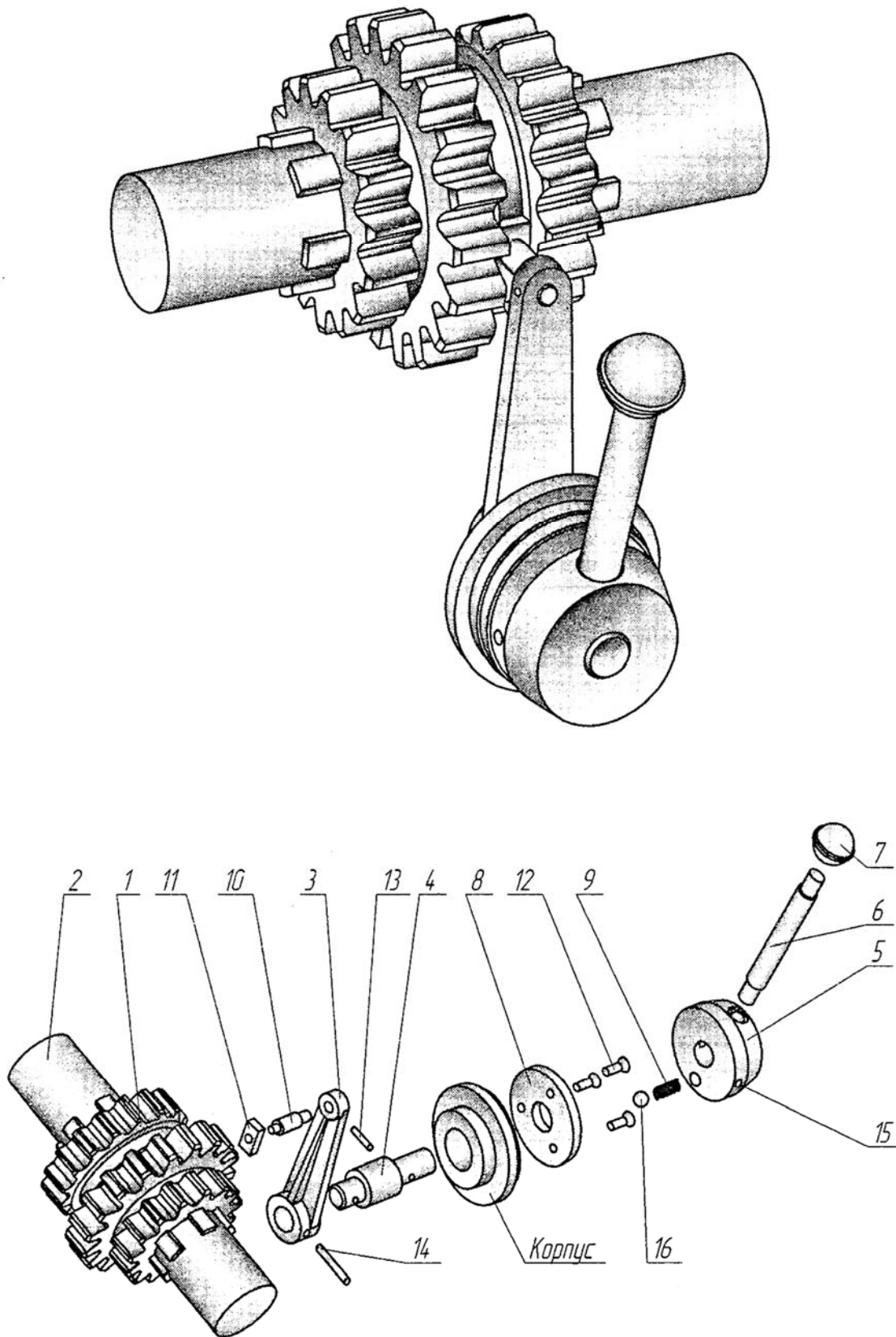
Рисунок 2.7 – Трехмерная модель механизма
