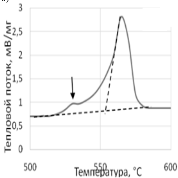
Рис. 1. Термограммы плавления эвтектических и заэвтектических силуминов, легированных медью: а – АК12 – 0,6 ат. % Cu; б – АК14 – 1 ат. % Cu; в – АК18 – 2 ат. % Cu
