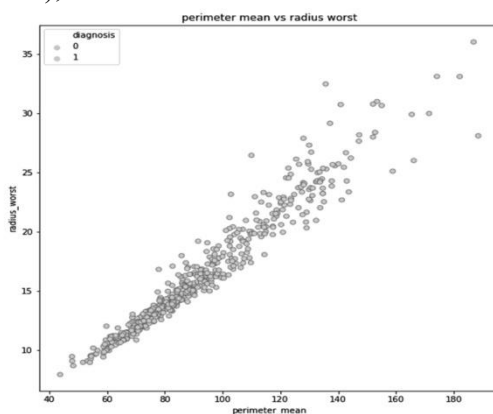
Рис. 2. Корреляция переменных perimeter mean и radius worst Fig. 2. Correlation of perimeter mean and radius worst variables
