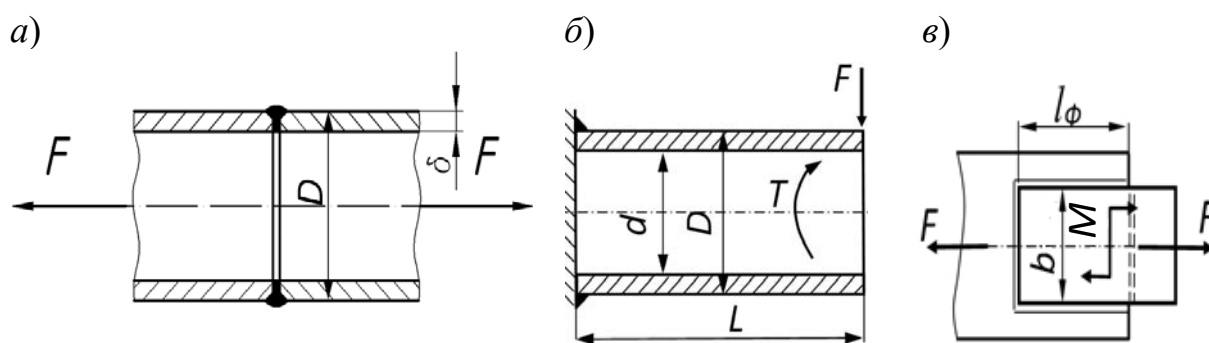
а – к задаче 1; б – к задачам 2 и 3; в – к задаче 4
