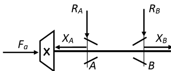
Рисунок 6 – Схема к задаче 4
