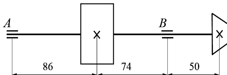
Рисунок 5 – Схема вала к задаче 4
