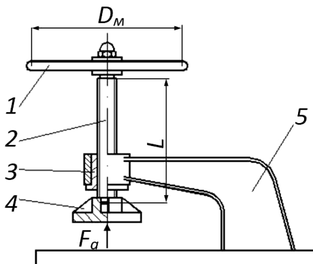
1 – маховик; 2 – винт; 3 – гайка; 4 – пятя; 5 – стойка
