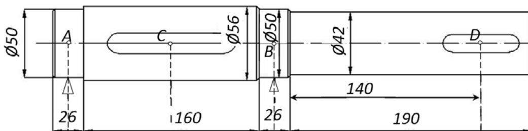
Рисунок 4 – Схема вала к задаче 1
