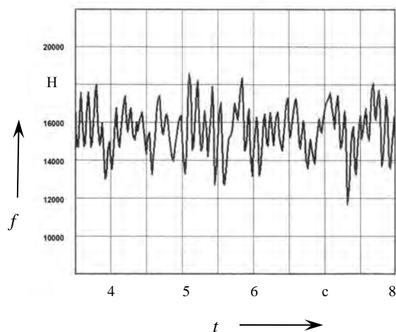
Рис. 4. Результаты моделирования действующих нагрузок при движении автомобиля по дороге без искусственной неровности
