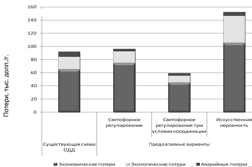
Рис. 12. Потери в дорожном движении по вариантам предлагаемых решений
