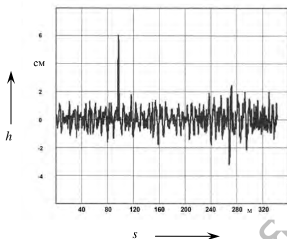
Рис. 2. Микронеровности покрытия исследуемого участка дороги
