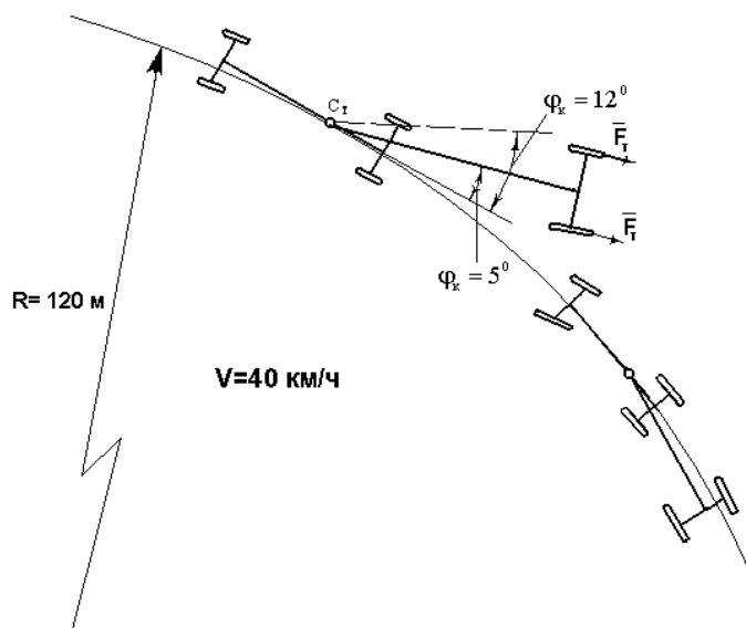
Рис. 1. Схематичное положение звеньев автопоезда при его торможении колесами оси полуприцепа
