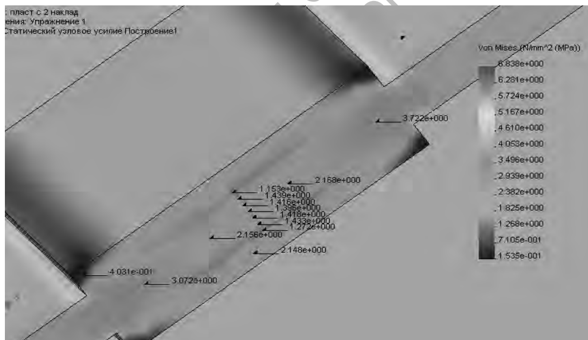
Рис. 4. Распределение нормальных напряжений в стыковом паяном соединении с двумя симметрично установленными накладками
