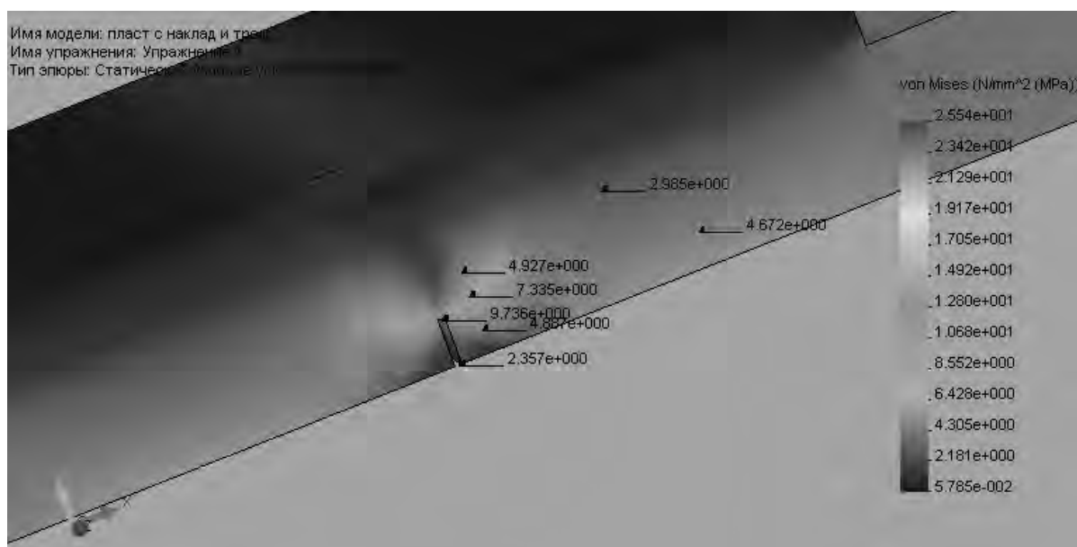
Рис. 3. Распределение интенсивности напряжений в паяном соединении с трещиной
