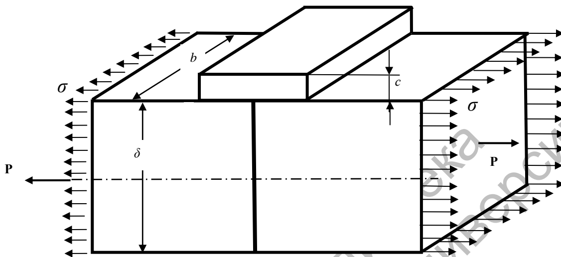
Рис. 1. Схема стыкового паяного соединения с накладкой
