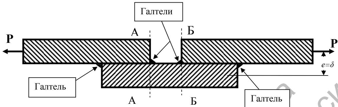
Рис. 6. Схема паяного соединения с односторонней накладкой, не имеющего стыкового шва
