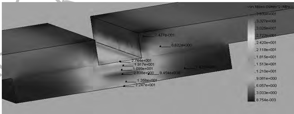
Рис. 7. Деформированная форма (а) и распределение интенсивности напряжений (б) в паяном соединении с односторонней накладкой при отсутствии стыкового шва
