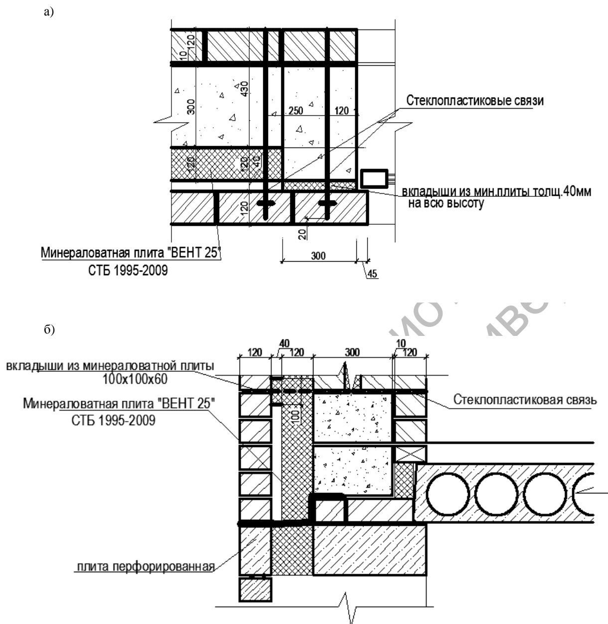
Рис. 5. Узлы примыкания оконных блоков к стенам: а – боковое примыкание оконного блока к стене; б – примыкание оконного блока сверху к стене
