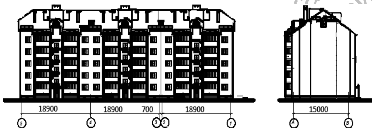
Рис. 1. Фасады теплоэнергоэффективного жилого здания
