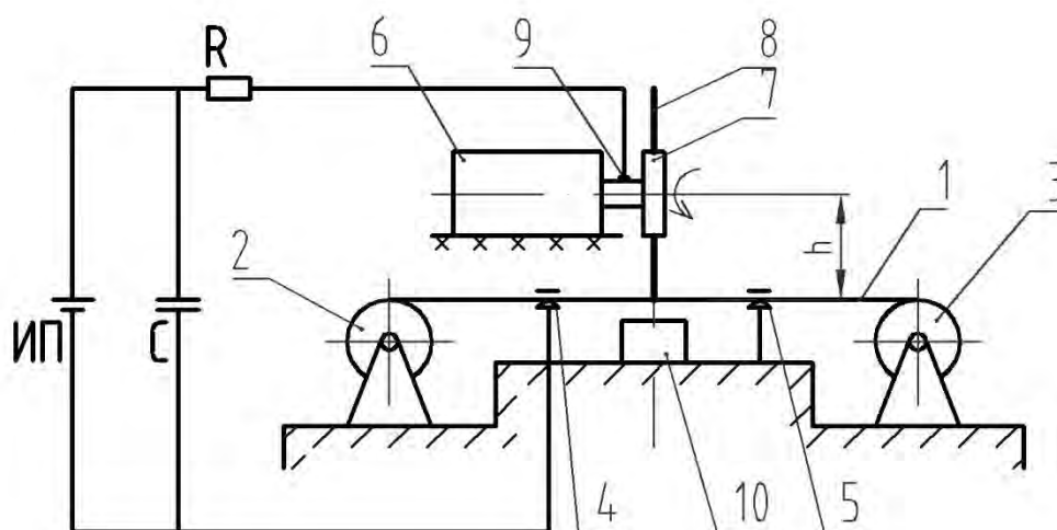
Рис. 2. Технологическая схема электроконтактной обработки поверхности проволочного инструмента с использованием электромеханического вибратора
