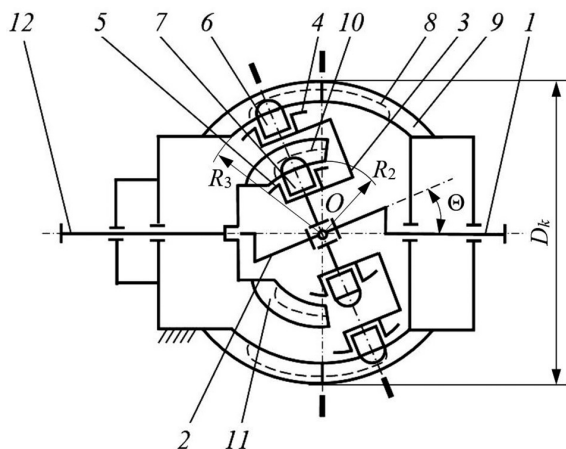
Рисунок 1 — Кинематическая схема сферической роликовой передачи с двухрядным сателлитом Figure 1 — Kinematic scheme of spherical roller transmission with double-row satellite
