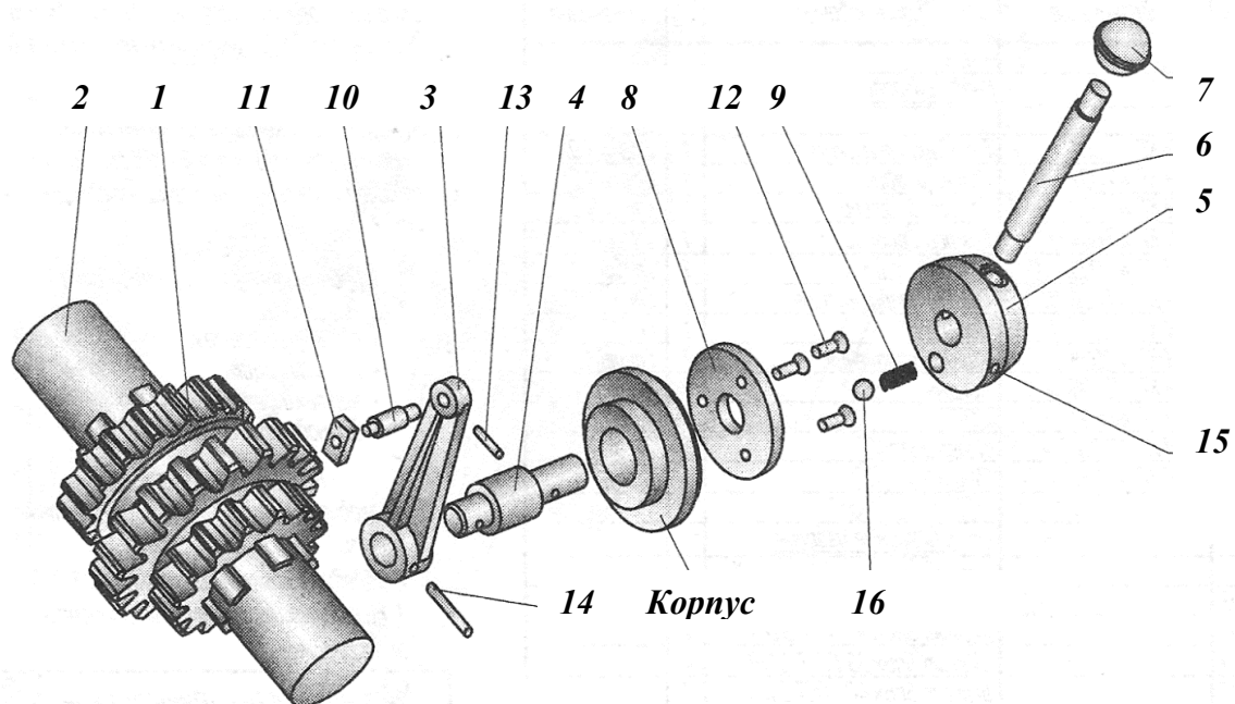
Рисунок 2.7 – Трёхмерная модель механизма
