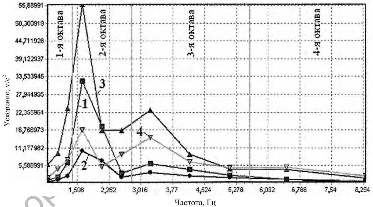
Рис. 7. Распределение вертикальных ускорений на сиденье водителя по третьоктавным полосам: 1 – асфальт, пассивная СП; 2 – асфальт, активная СП; 3 – грунтовая дорога, пассивная СП; 4 – грунтовая дорога, активная СП
