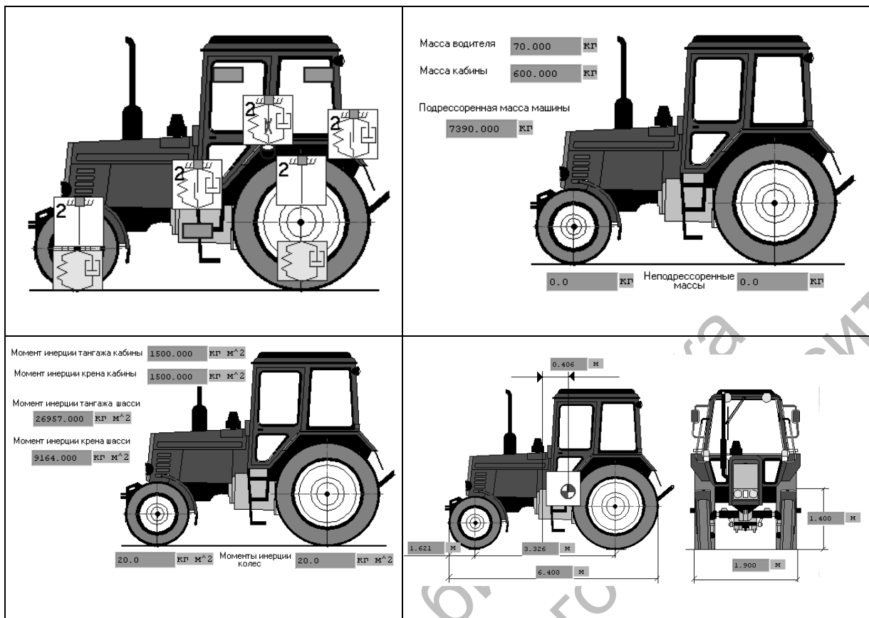
Рис. 4. Основные параметры колесного трактора
