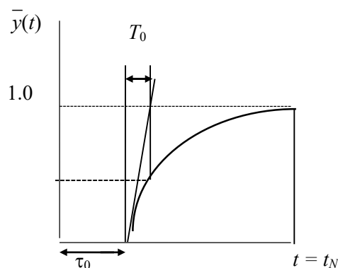
Рисунок 9.1 – Экспериментальная кривая разгона объекта управления в относительных единицах
