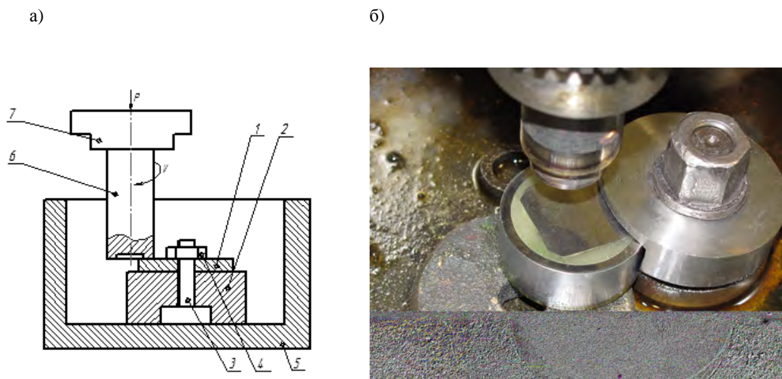
Рис. 4. Схема (а) и фотография (б) установки для проведения испытаний износостойкости образцов: 1 – образец; 2 – подставка; 3 – шпилька; 4 – фиксирующая гайка; 5 – емкость; 6 – контроллер; 7 – патрон
