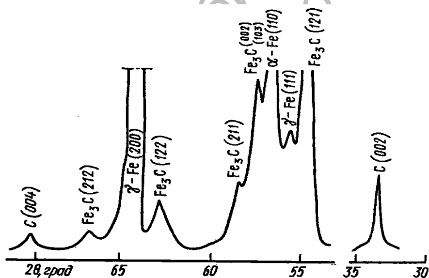
Рис. 2. Рентгенограмма зоны оплавления чугуна после обработки непрерывным CO 2 -лазером
