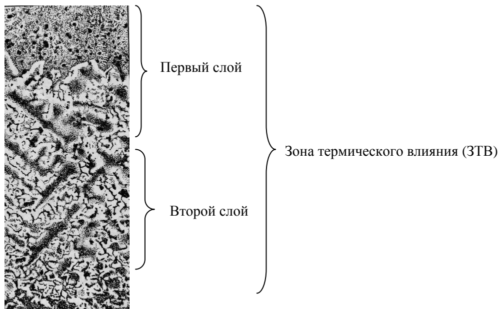
Рис. 1. Микроструктура чугуна после обработки непрерывным CO 2 -лазером (×300)
