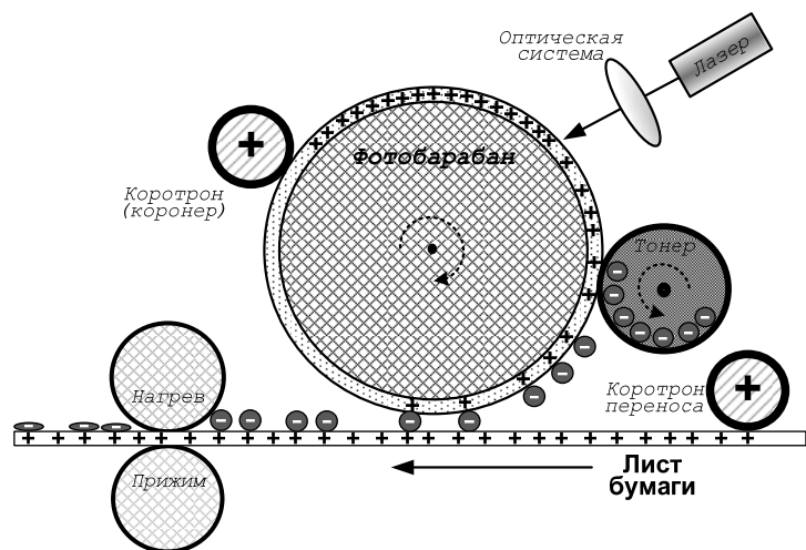
Рисунок 8.1 – Функциональная схема работы лазерного принтера
