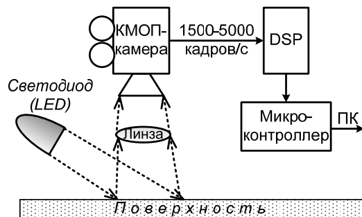
Рисунок 5.2 – Схема работы оптосенсорной мыши
