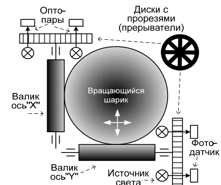
Рисунок 5.1 – Принцип действия опто-механической мыши
