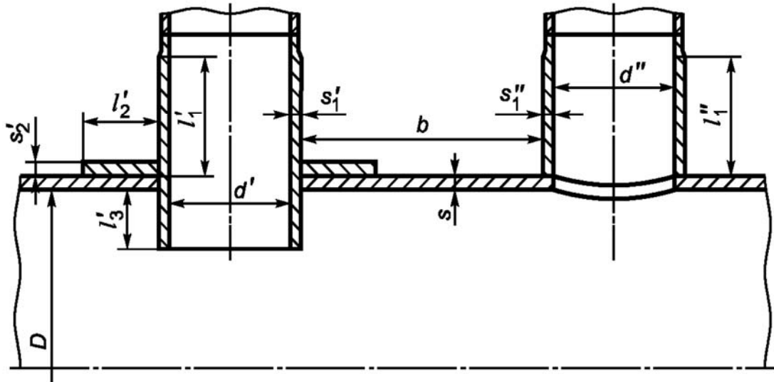
Рисунок 3.3 – Укрепление взаимовлияющих отверстий
