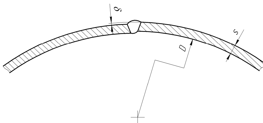
Рисунок 4.1 – Смещение кромок в продольном шве
