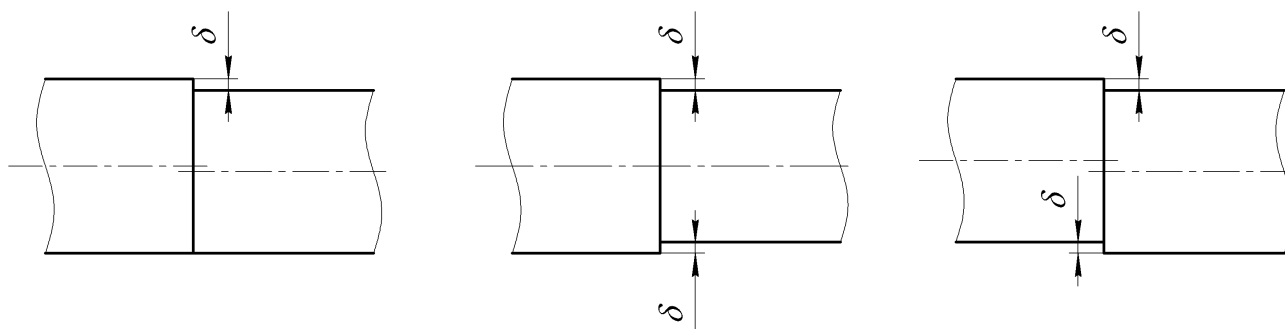
Рисунок 4.2 – Смещение кромок в кольцевых швах
