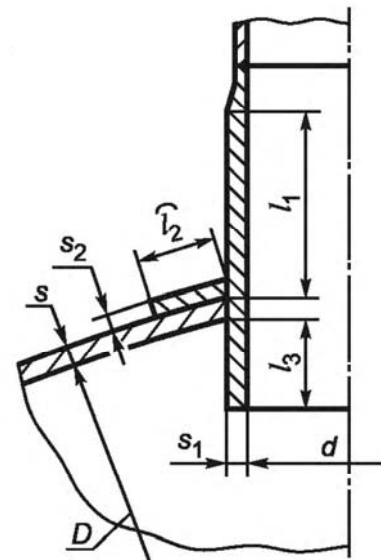
Рисунок 3.2 – Укрепление отверстий накладным кольцом при наличии проходного штуцера
