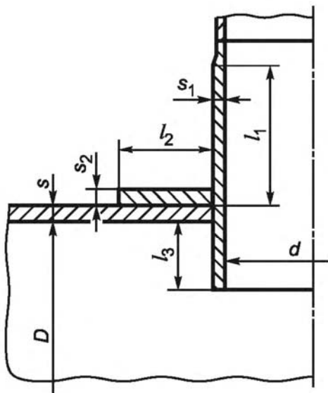
Рисунок 3.2 – Укрепление отверстий накладным кольцом при наличии проходного штуцера
