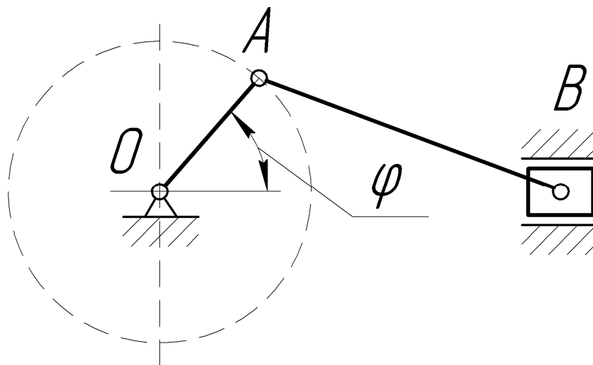
Рисунок 1.1 – Кривошипно-ползунный механизм
