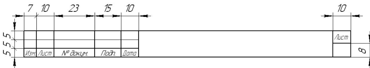
Рисунок 12 – Основная надпись по ГОСТ 2.104–68 (форма 2а)
