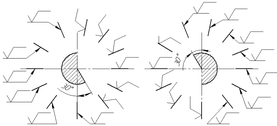
Рисунок 16 – Расположение обозначения шероховатости поверхности в зависимости от ее расположения
