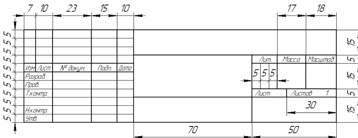
Рисунок 11 – Основная надпись по ГОСТ 2.104–68 (форма 1)
