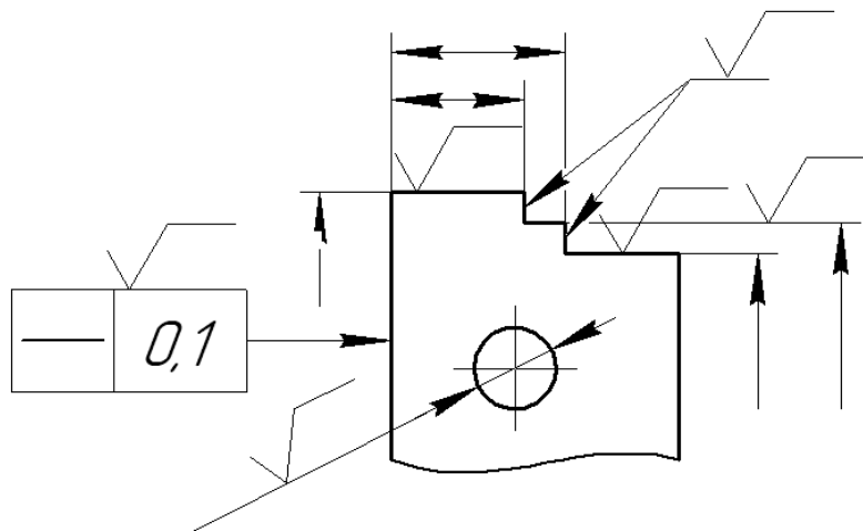
Рисунок 15 – Расположение обозначения шероховатости поверхности
