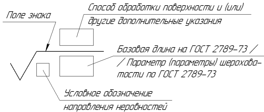
Рисунок 14 – Обозначение шероховатости поверхности
