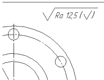
Рисунок 17 – Обозначение неуказанной шероховатости поверхности
