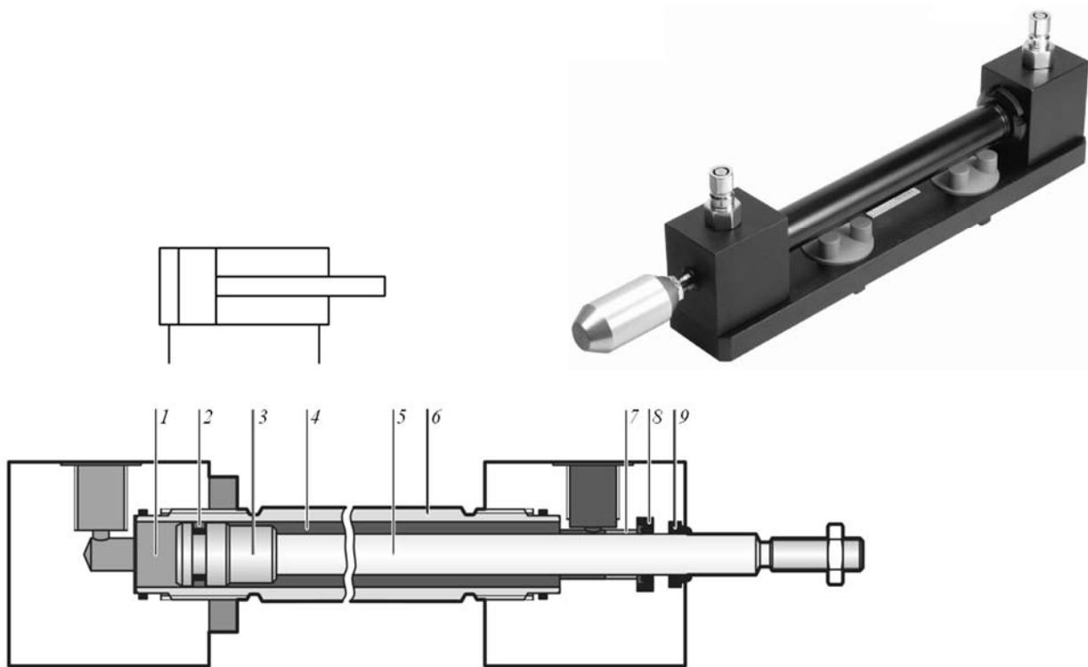
1 – бесштоковая полость; 2 – уплотнение на поршне; 3 – поршень; 4 – штоковая полость; 5 – шток гидроцилиндра; 6 – гильза цилиндра; 7 – направляющая втулка; 8 – уплотнение штока; 9 – пыльник
