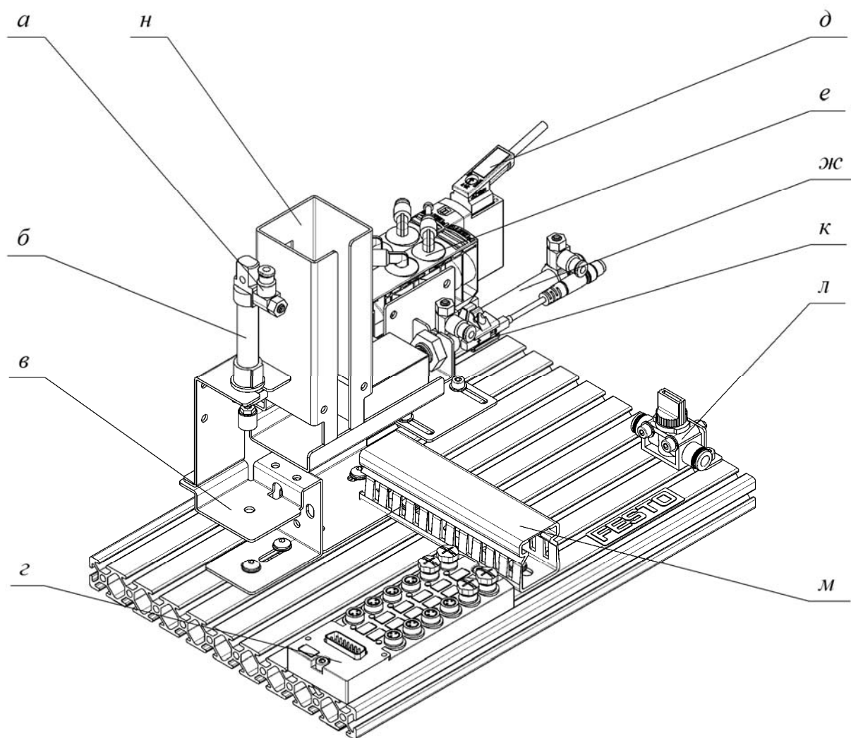
Рисунок 6.1 – Внешний вид станции стекового накопителя
