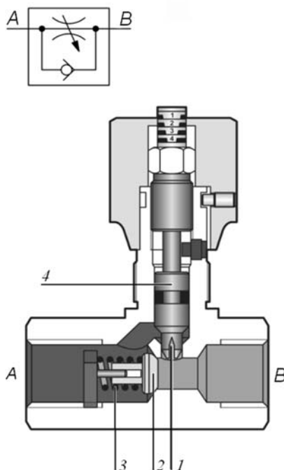
Рисунок 2.1 – Дроссель FESTO 152843
