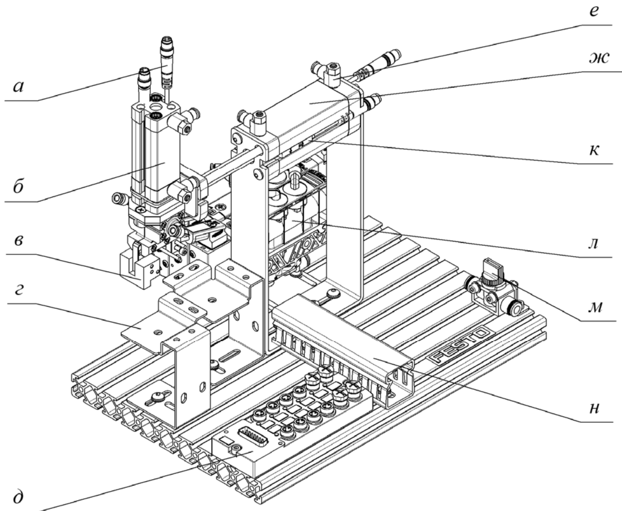
Рисунок 7.2 – Внешний вид станции манипулятора
