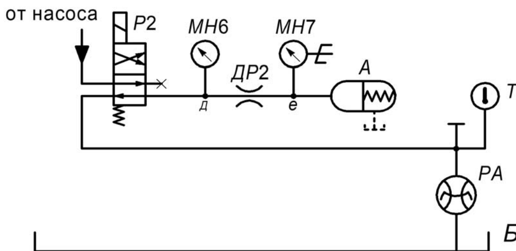
Рисунок 4.2 – Схема объекта испытаний
