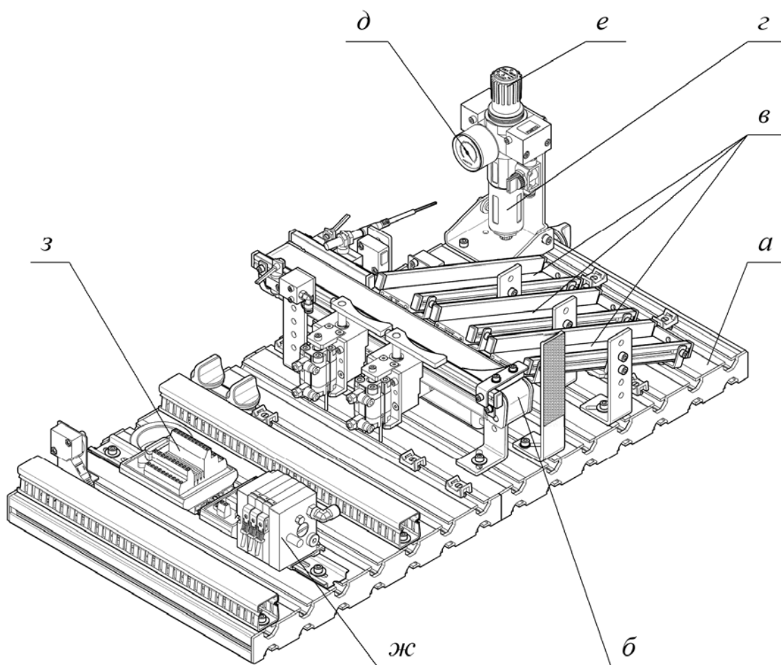
Рисунок 8.1 – Общий вид станции сортировки
