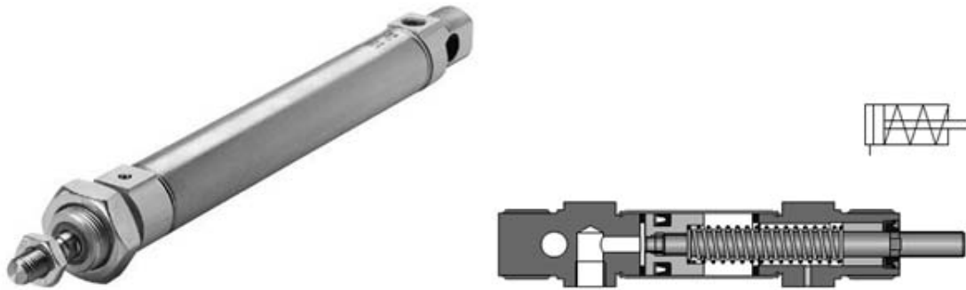
Рисунок 5.1 – Пневматический цилиндр одностороннего действия с пружинным возвратом
