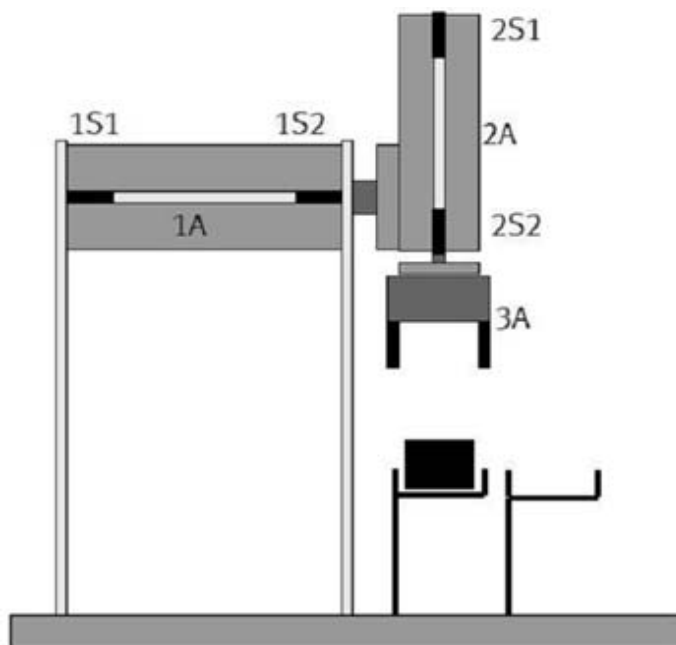
Рисунок 7.1 – Схематическое изображение станции манипулятора
