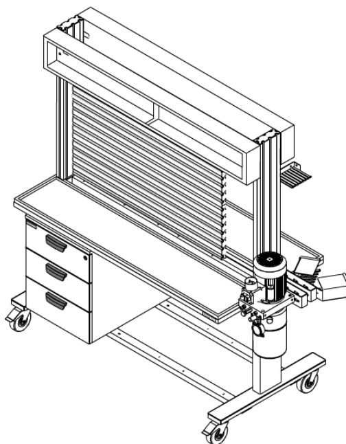
Рисунок 1.6 – Лабораторный стенд
