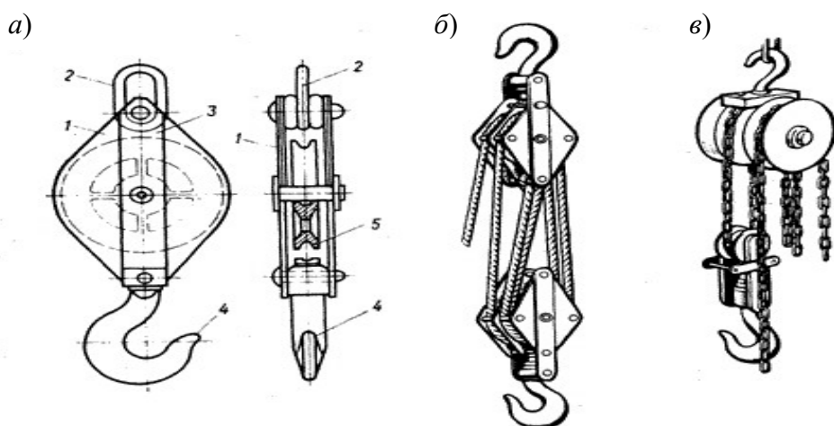
а – блок; б – полиспаст; в – таль; 1 – щека; 2 – проушина; 3 – обойма (скоба); 4 – крюк; 5 – ролик
