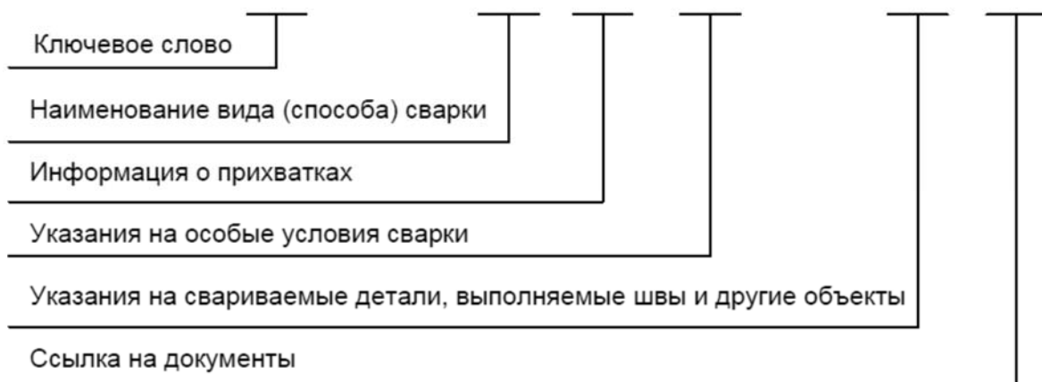
Рисунок 6.1 – Схема содержания сварочного перехода
