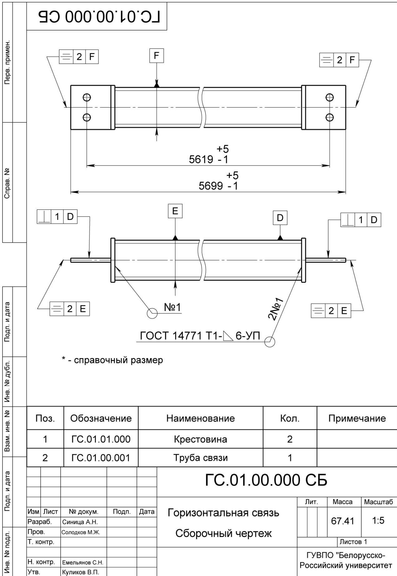
Рисунок 6.3 – Чертеж горизонтальной связи
