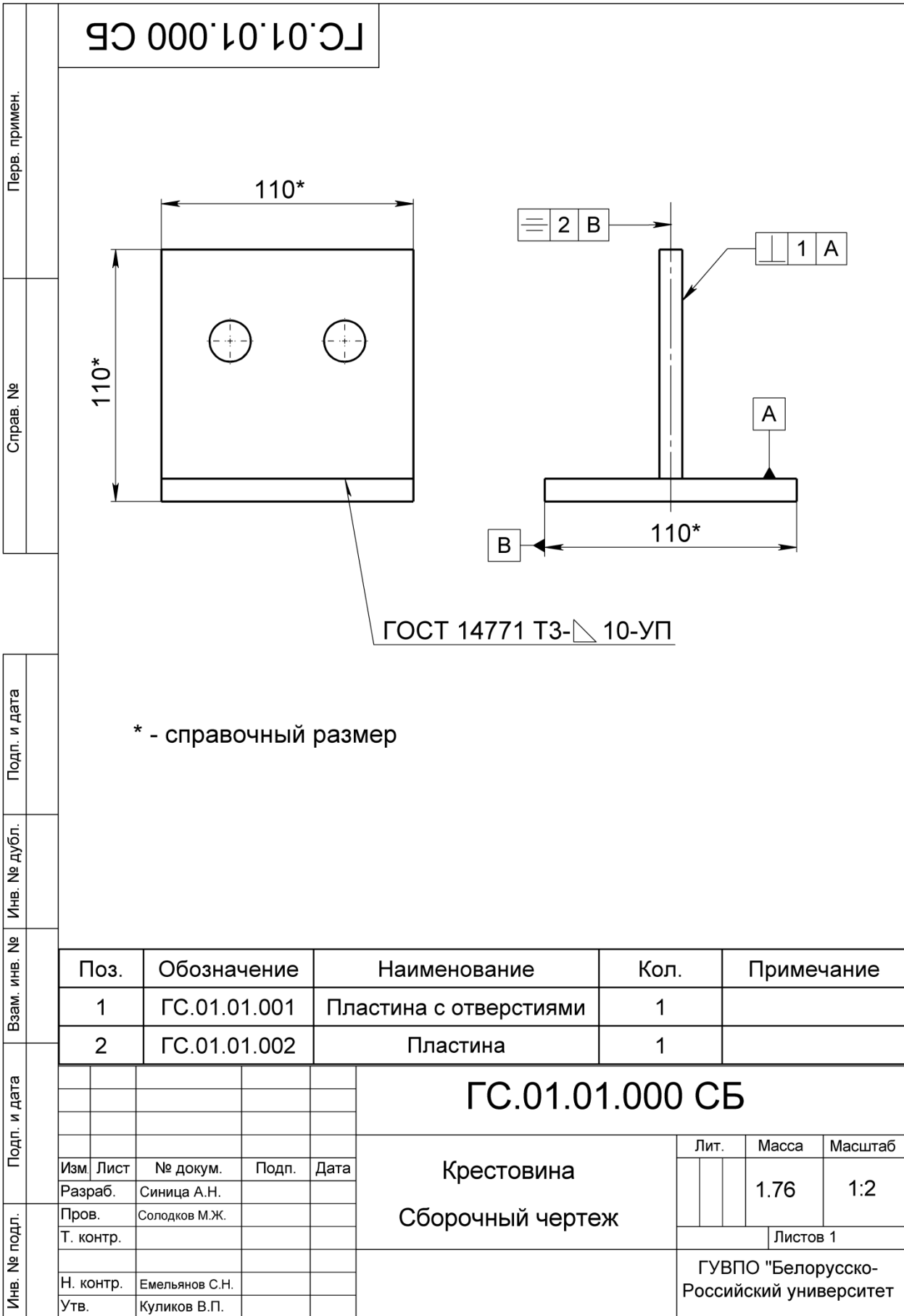
Рисунок 6.4 – Крестовина. Сборочный чертеж
