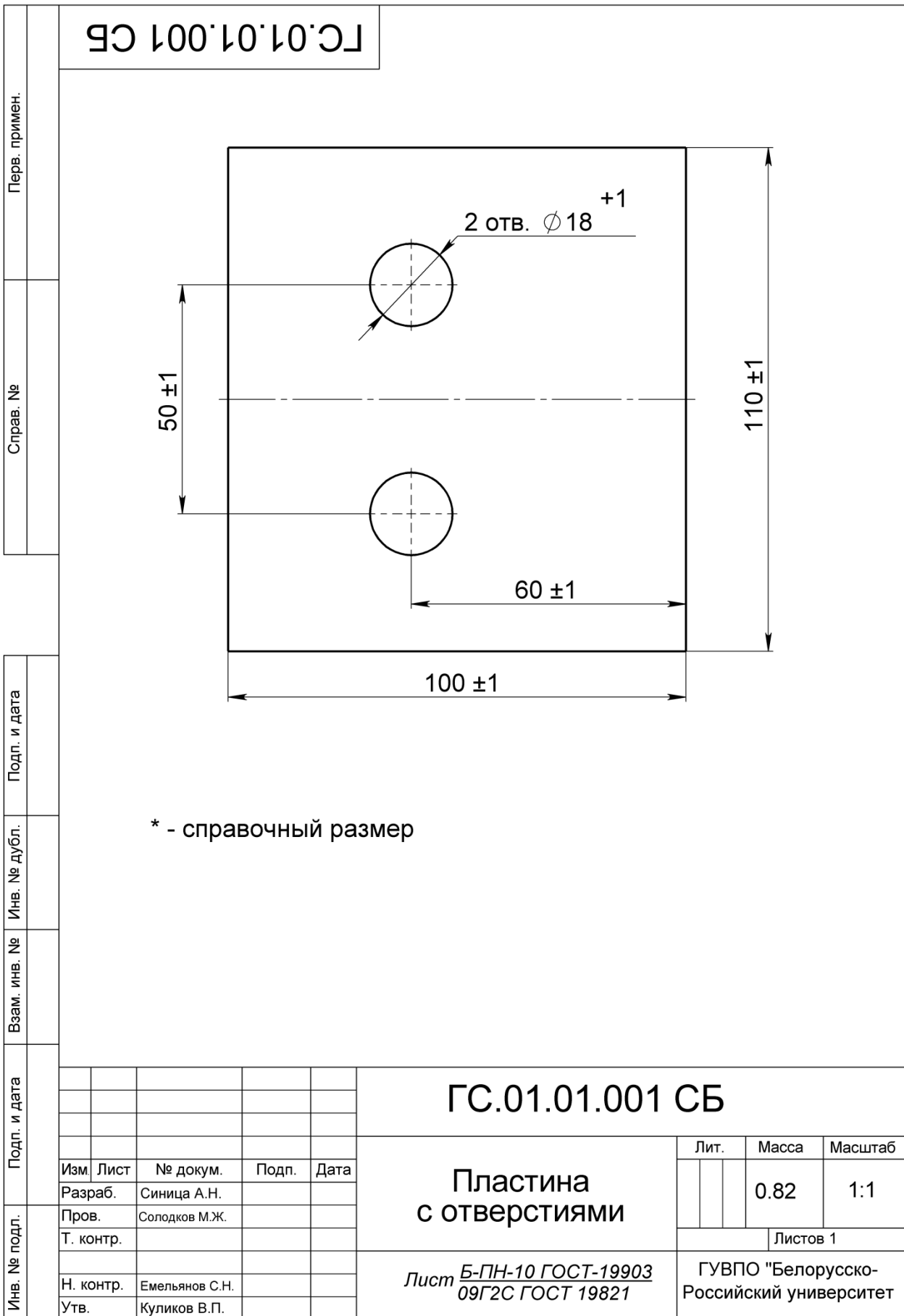
Рисунок 6.6 – Чертеж пластины с отверстиями
