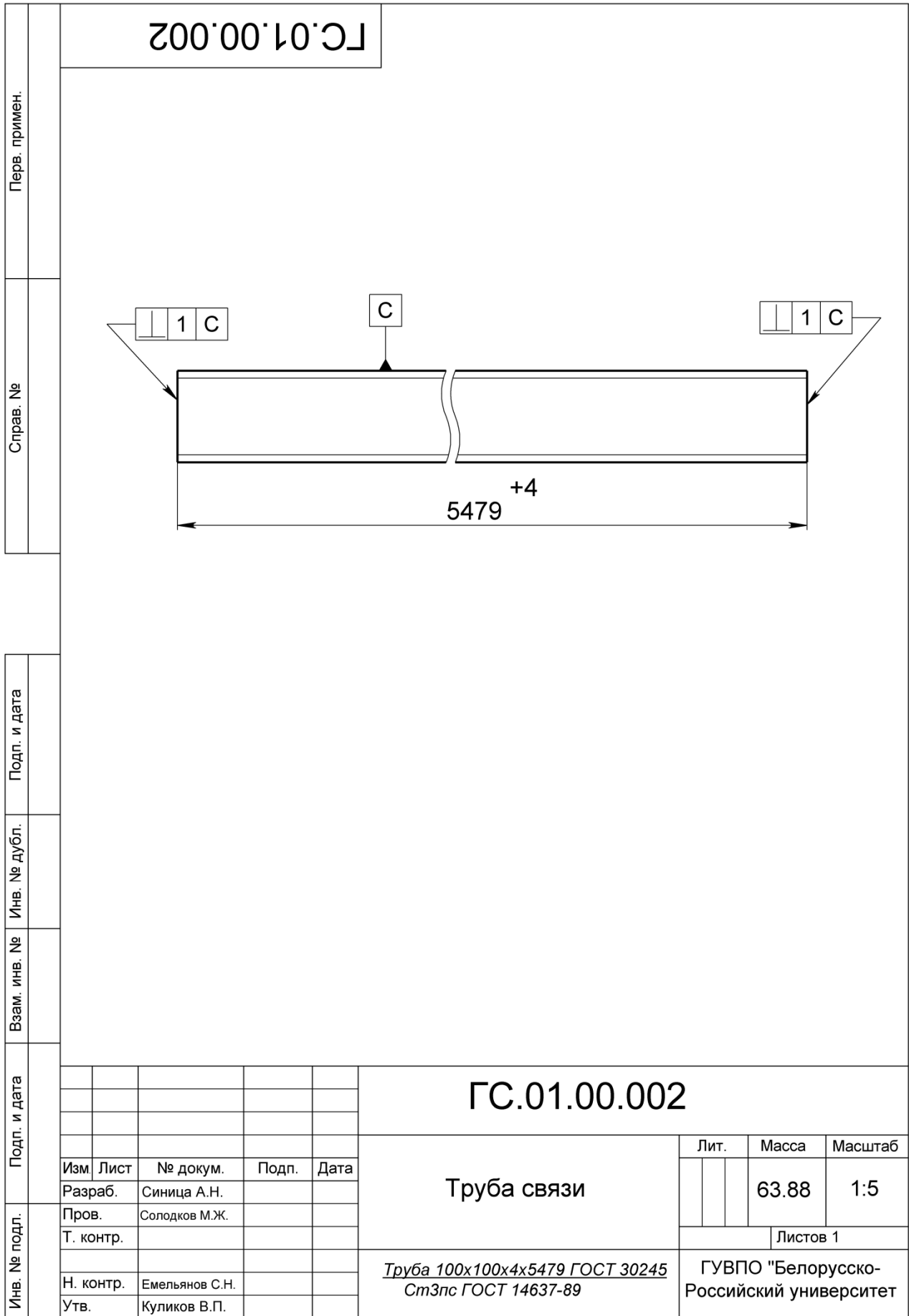
Рисунок 6.5 – Чертеж трубы
