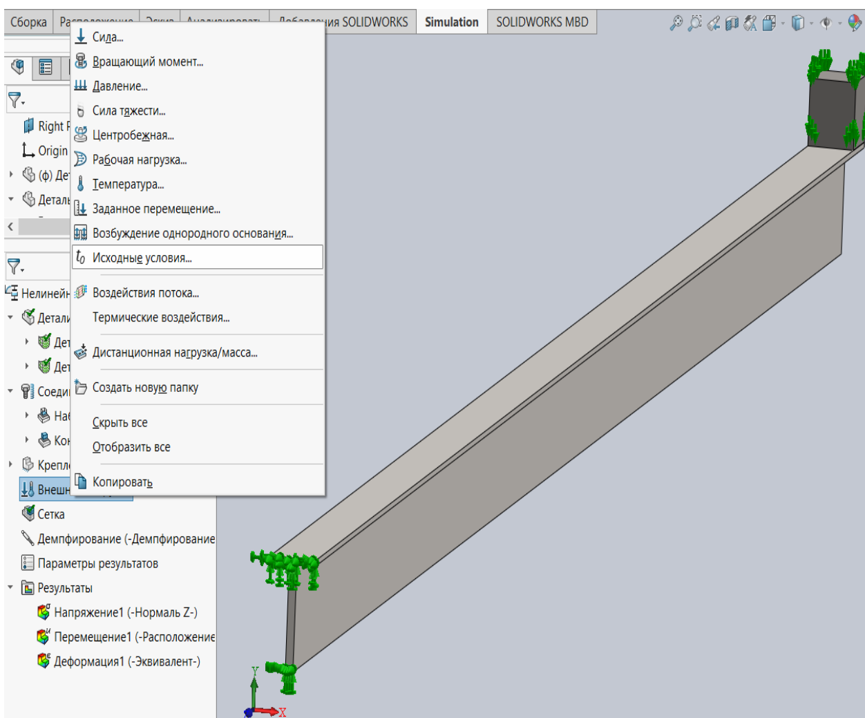
Рисунок 4.7 – Задание Исходных условий в момент соприкосновения груза с балкой
