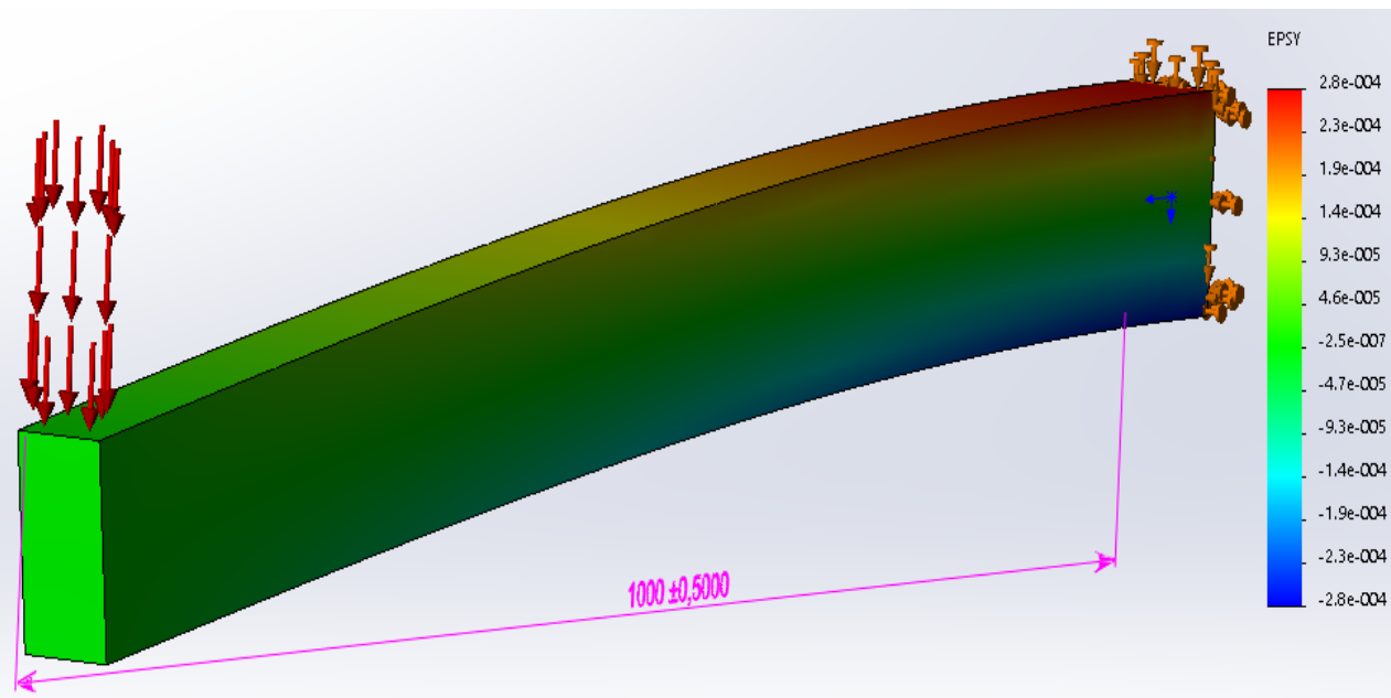
Рисунок 2.8 – Распределение относительных линейных деформаций \epsilon_y в направлении, перпендикулярном поперечному сечению балки
