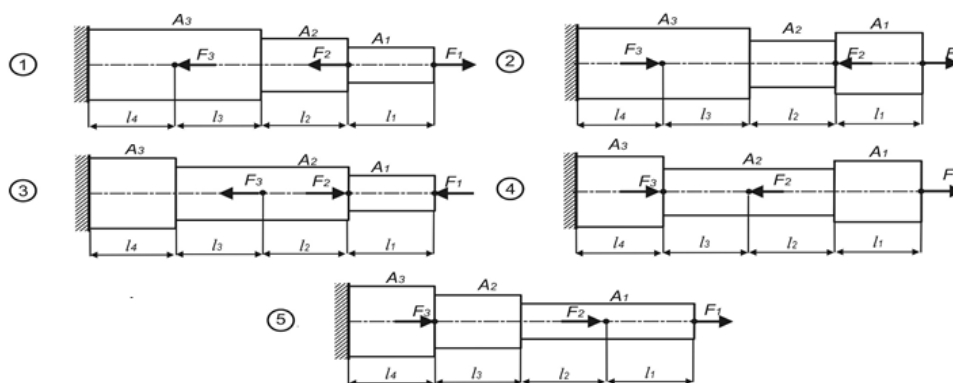
Рисунок 5.1 – Варианты расчетных схем бруса
