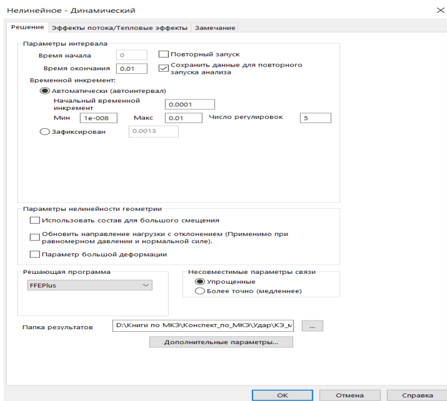
Рисунок 4.5 – Диалоговое окно настройки расчетной части
