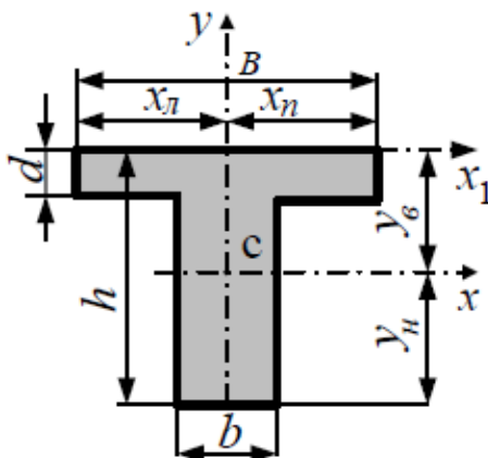
Рисунок 4.2 – Форма поперечного сечения рассматриваемой балки
