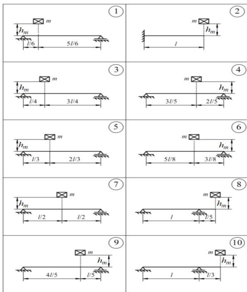
Рисунок 5.2 – Расчетные схемы для анализа поперечного удара по балке
