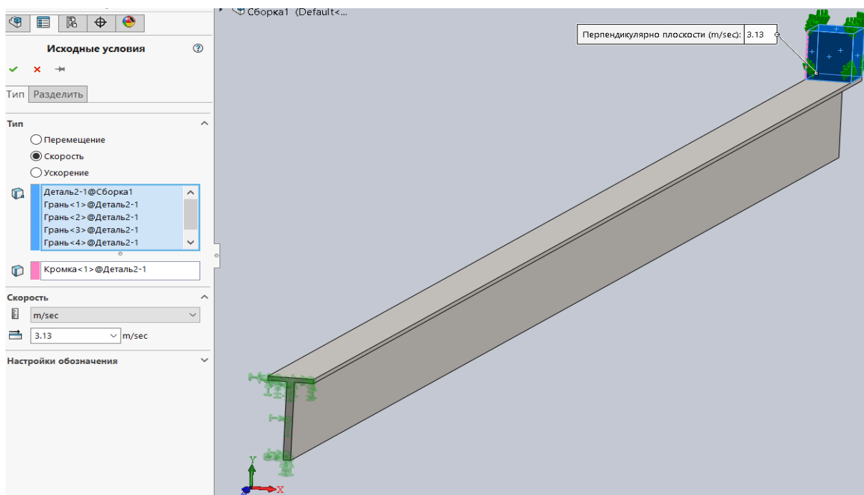
Рисунок 4.8 – Исходные условия для разработанной конечно-элементной модели
