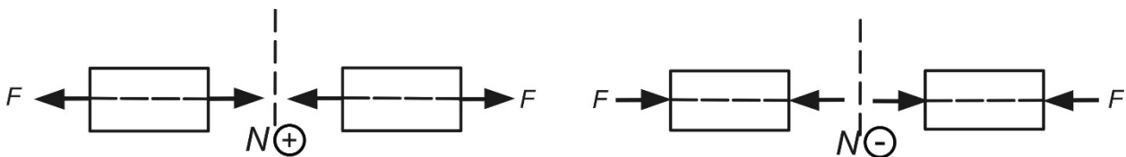
Рисунок 1.2 – Правило знаков для продольных сил
