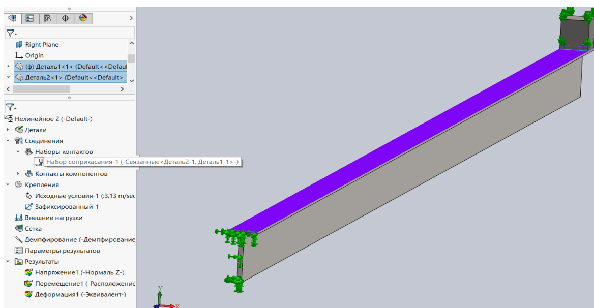
Рисунок 4.6 – Условия соединения в зоне контакта верхней поверхности балки и груза
