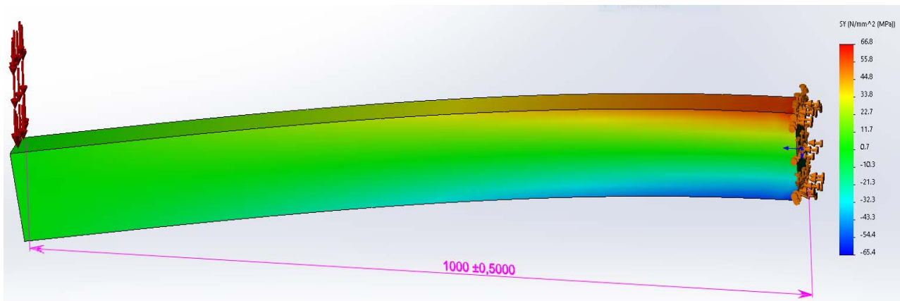
Рисунок 2.6 – Распределение нормальных напряжений в направлении, перпендикулярном поперечному сечению балки
