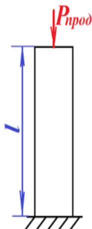
Рисунок 3.1 – Расчетная схема для определения критической силы центрально-сжатой стойки
