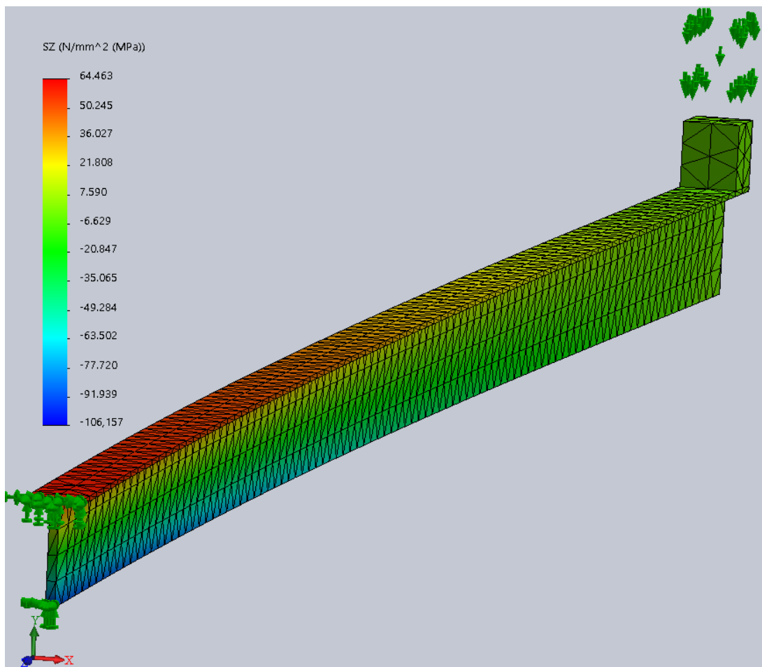
Рисунок 4.11 – Распределение нормальных напряжений по наружной поверхности балки в момент наибольшего деформирования ее
