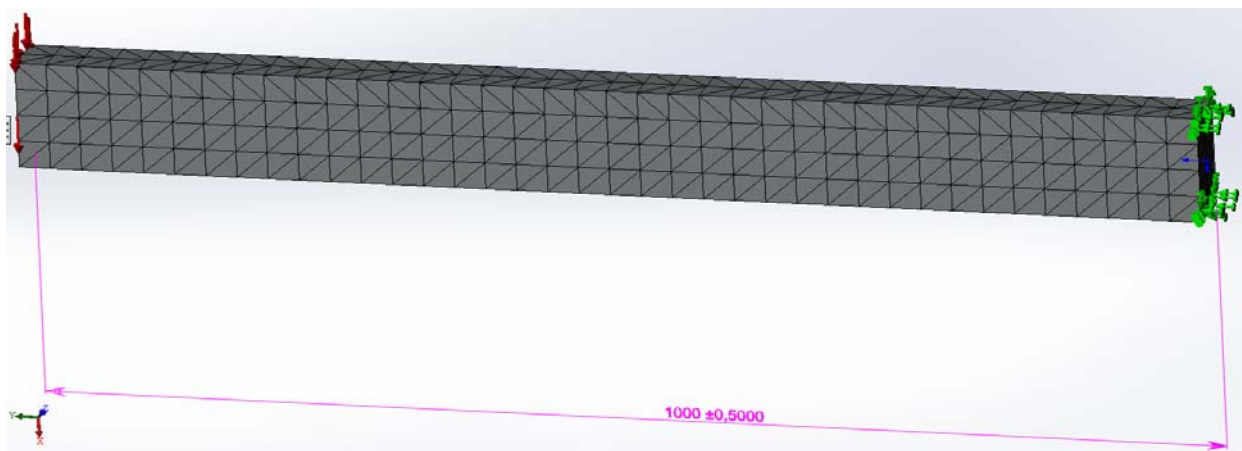
Рисунок 2.4 – Конечно-элементная модель консольно-закрепленной балки, нагруженной на свободном конце поперечной нагрузкой, равномерно распределенной по плоскости торца
