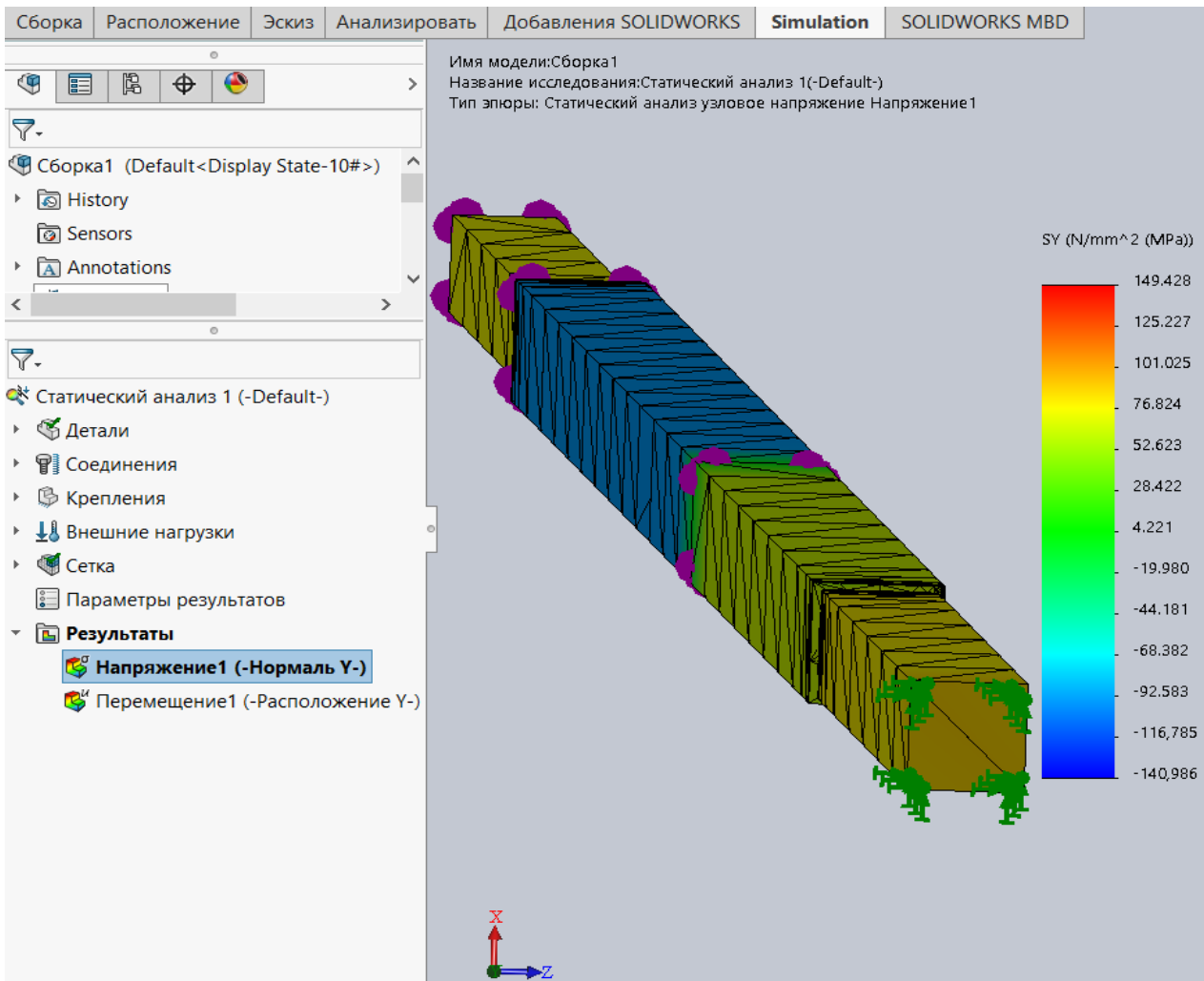
Рисунок 1.7 – Эпюра нормальных напряжений рассматриваемого ступенчатого бруса
