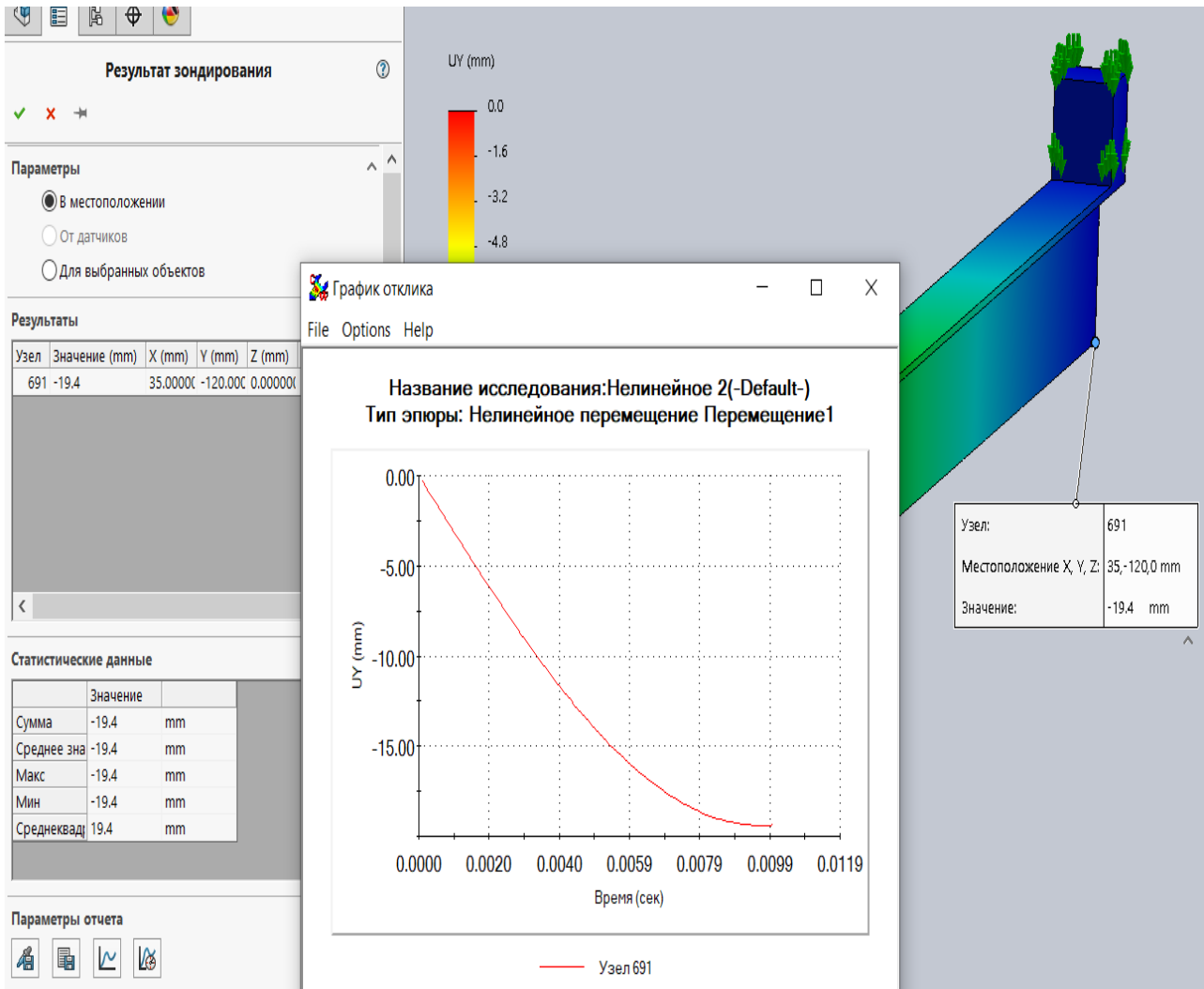
Рисунок 4.13 – График прогиба балки в зоне падения груза за активную фазу удара
