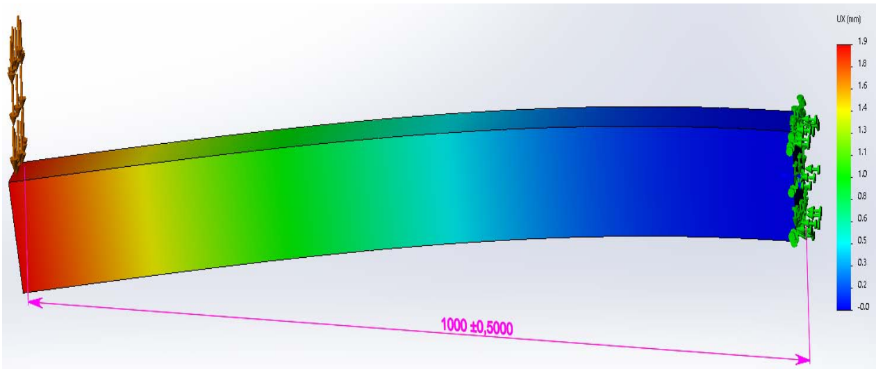
Рисунок 2.7 – Перемещения точек поверхности балки в вертикальном направлении
