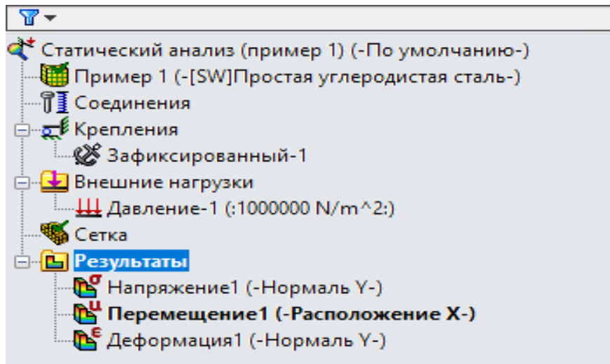
Рисунок 2.5 – Меню пункта «Результаты» после проведения расчета
