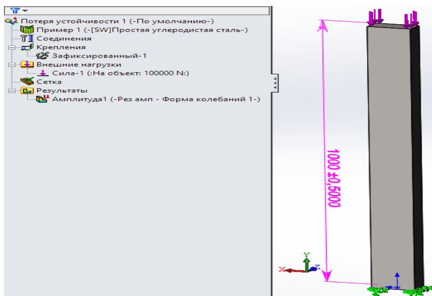
Рисунок 3.2 – Модель расчета продольно-сжатого стержня усилием 100000 Н, прямоугольного поперечного сечения 50×100 мм, длиной 1000 мм, нижний край которого жестко защемлен, и дерево менеджера Simulation применительно к расчетам по проверке потери устойчивости
