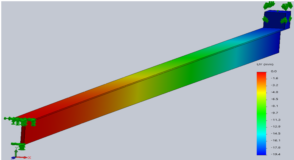
Рисунок 4.10 – Максимальный прогиб балки в процессе поперечного удара
