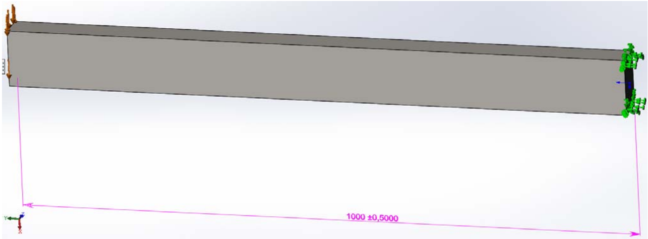
Рисунок 2.3 – Модель исследуемого объекта с изображением действующей нагрузки и условиями закрепления
