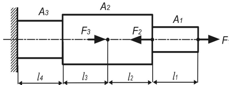
Рисунок 1.1 – Расчетная схема анализируемого бруса
