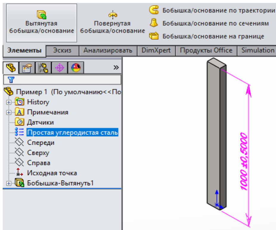
Рисунок 2.2 – Твердотельная модель стержня, длина которого составляет 1000 мм, состоящего из материала «простая углеродистая сталь»
