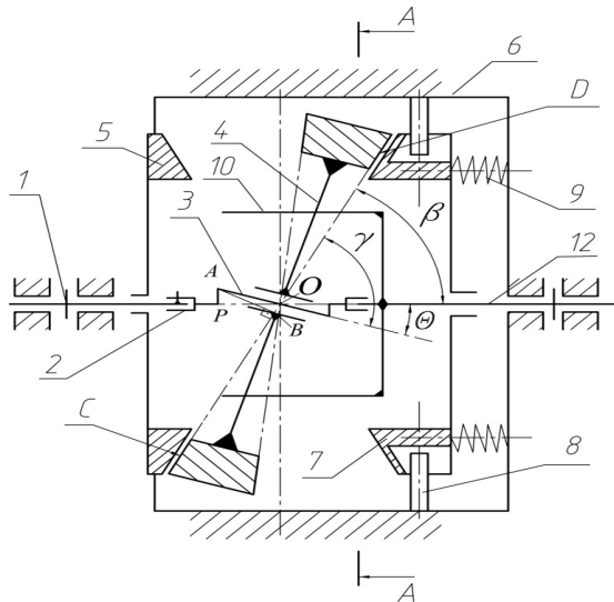
Рис. 1. Структурная схема прецессионной передачи типа К-Н-V фрикционного типа
