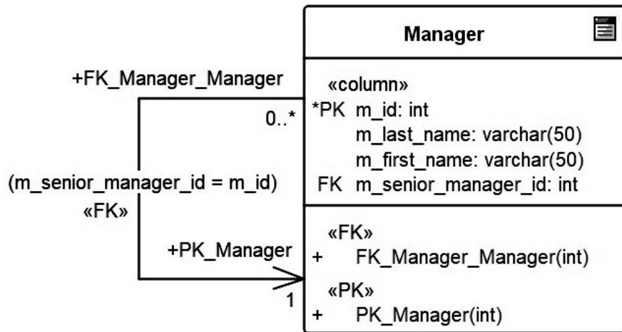
Рисунок 3.8 – Рекурсивная связь
