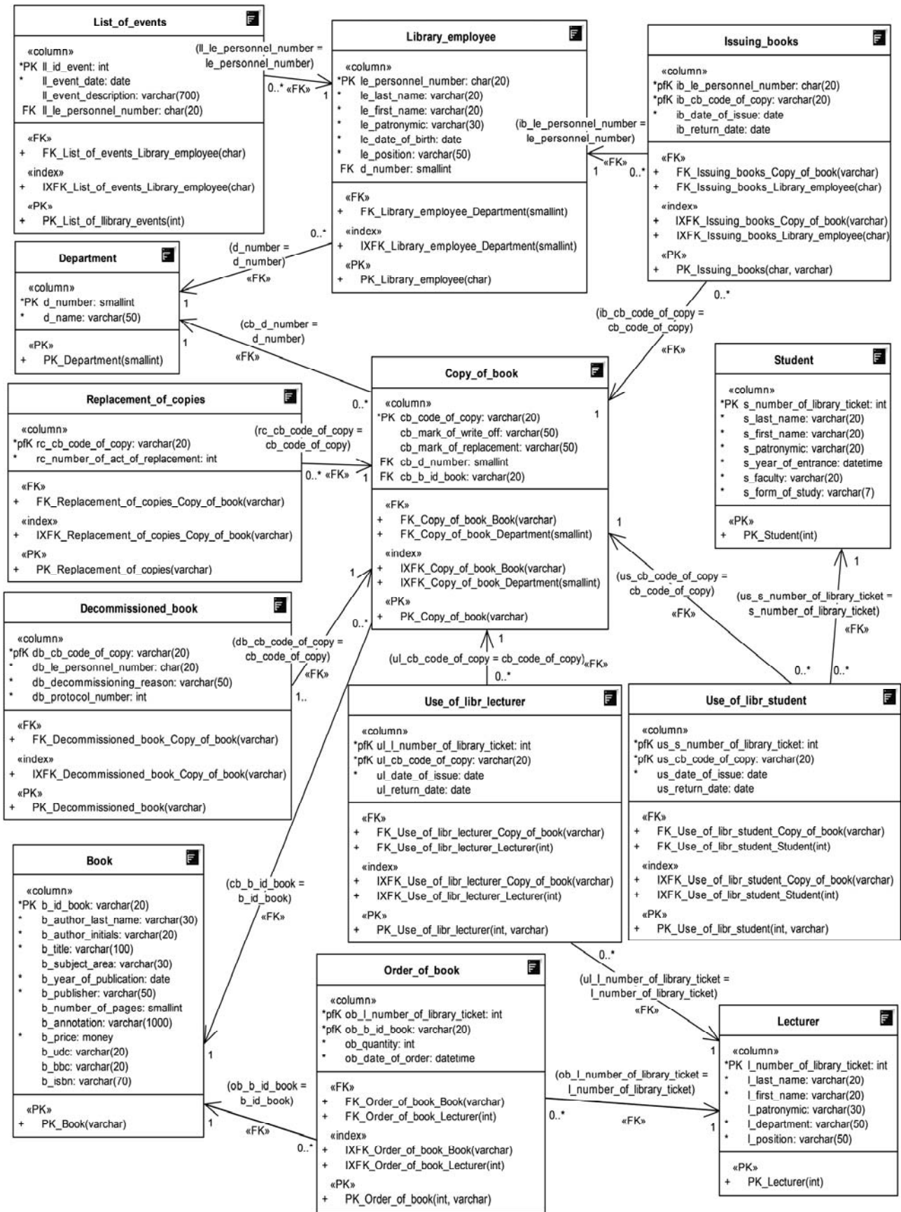
Рисунок 3.10 – Информационная модель
