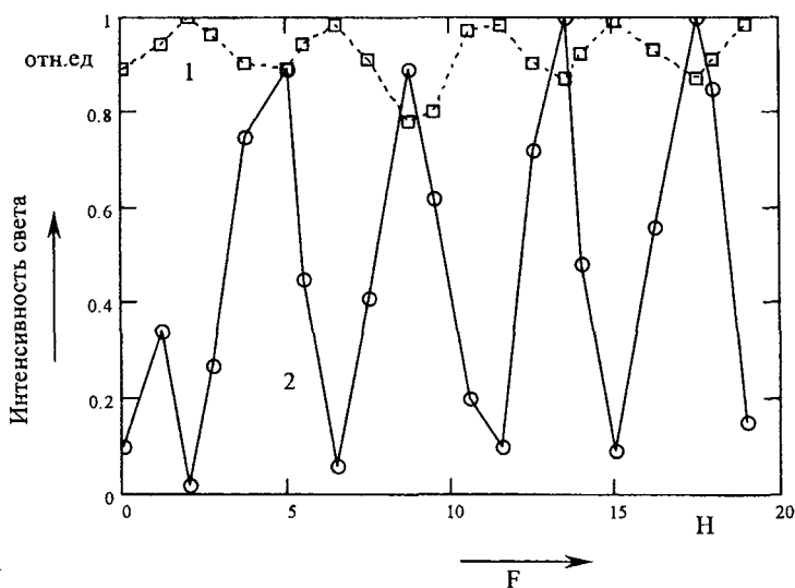
Рис. 5. Залежність сигналу на виході одномодового волоконного світловода для випадку, коли напрямлення дії сили збігається з площиною поляризації возбуждаючого світловода
