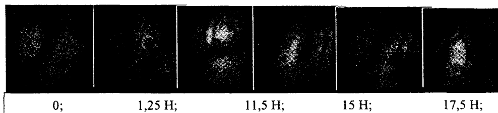
Рис. 3. Перестройка модовой структуры двухмодового волоконного световода при различной величине бокового сжатия
