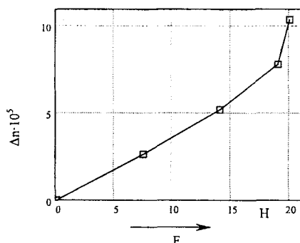
Рис. 2. Зависимость изменения эффективного показателя преломления моды двухмодового волоконного световода от величины силы, приложенной к световоду
