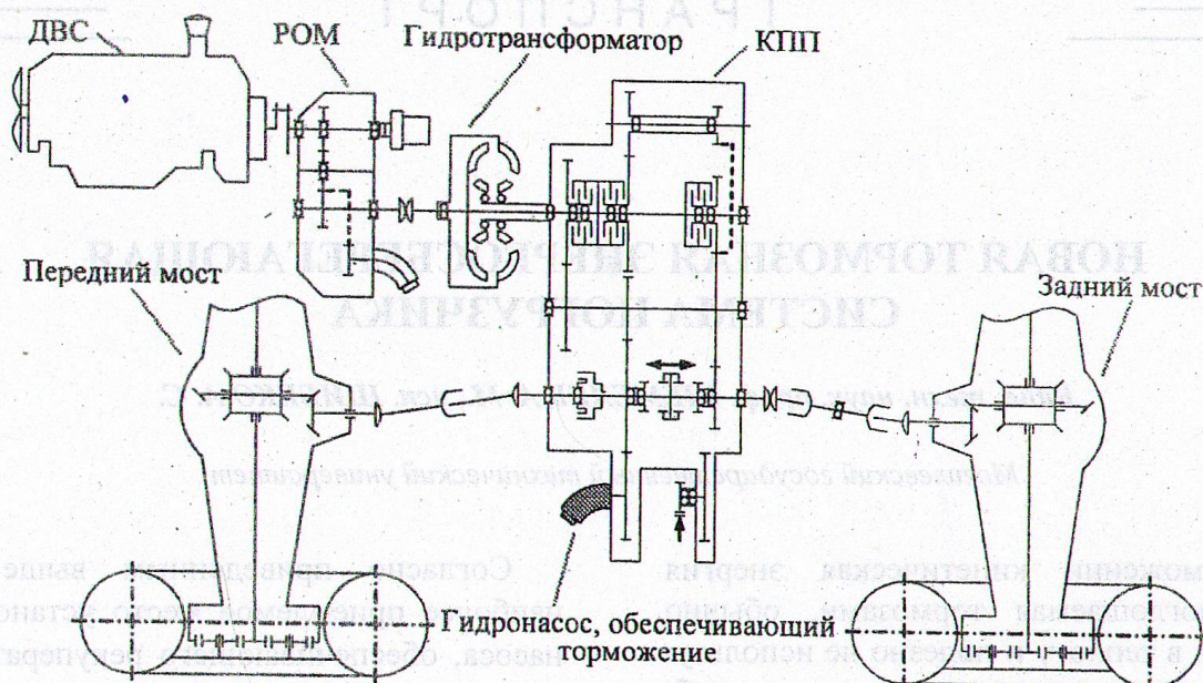
Рис. 1. Кинематическая схема погрузчика ТО-18Б
