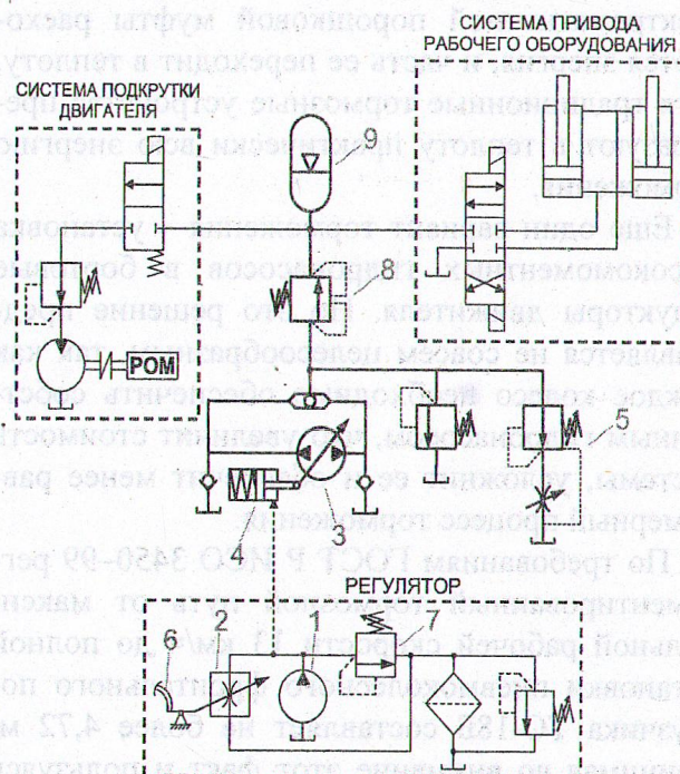
Рис. 2. Гидросхема системы торможения подкрутки с регулируемым гидронасосом
