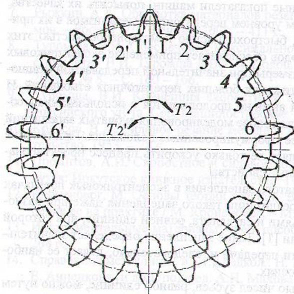
Рис. 1. Схема модифицированного зубчатого зацепления ( z_1 = 21 )
