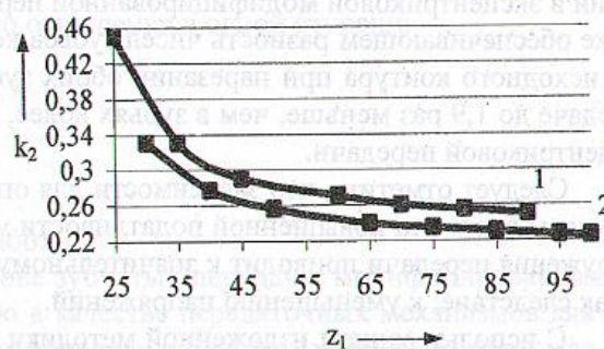
Рис. 4. Зависимости коэффициентов, учитывающих распределение нагрузки k_1 (а) и k_2 (б), от числа зубьев сателлита: 1 — n_z = 2 ; 2 — n_z = 3
