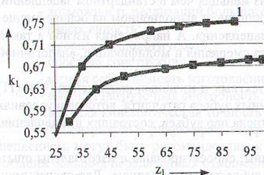
Рис. 4. Зависимости коэффициентов, учитывающих распределение нагрузки k_1 (а) и k_2 (б), от числа зубьев сателлита: 1 — n_z = 2 ; 2 — n_z = 3
