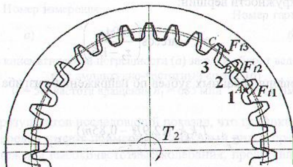
Рис. 3. Схема для силового анализа ( z_1 = 50 ):
