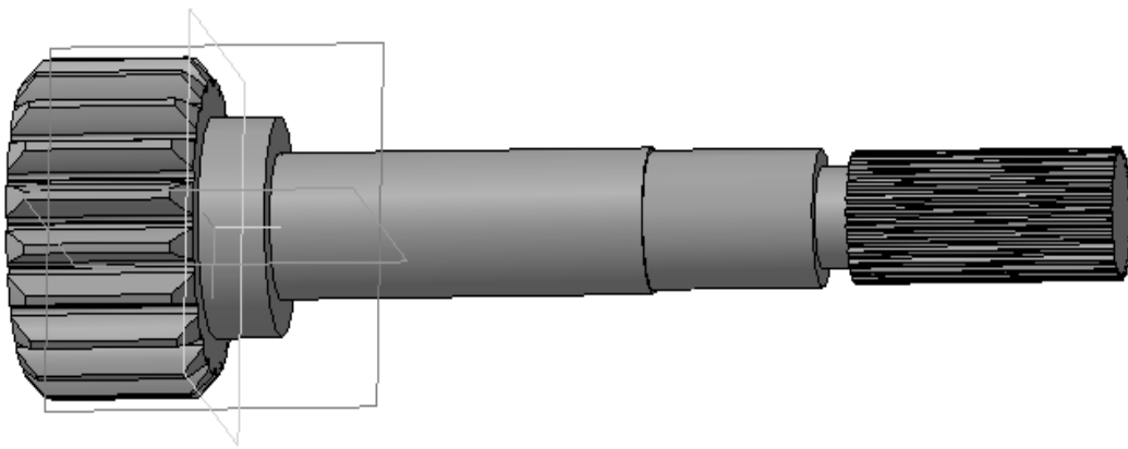
Рисунок 3.2 – Вал-шестерня
