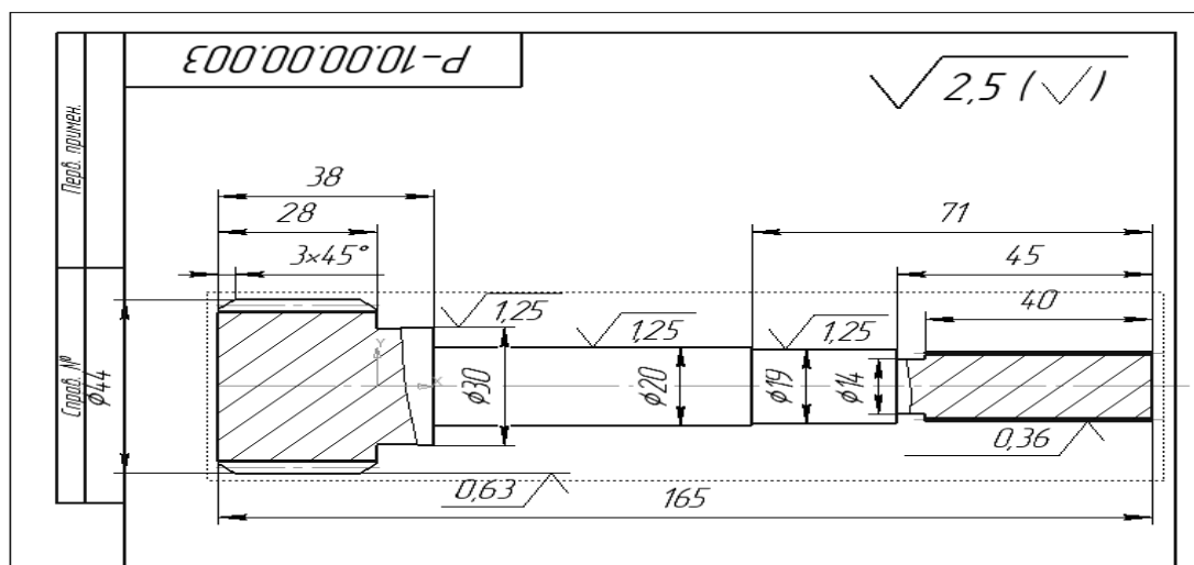
Рисунок 5.1 – Вал-шестерня
