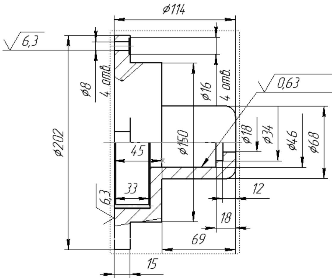
Рисунок 5.2 – Корпус
