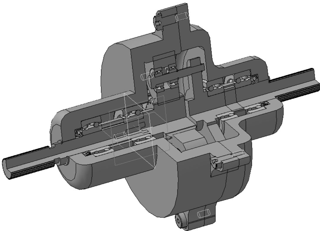
Рисунок 4.1 – Пример зубчатого планетарного редуктора
