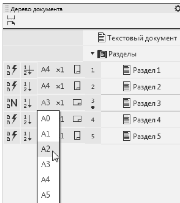
Рисунок 1.8 – Смена параметров объекта в Дереве документа
