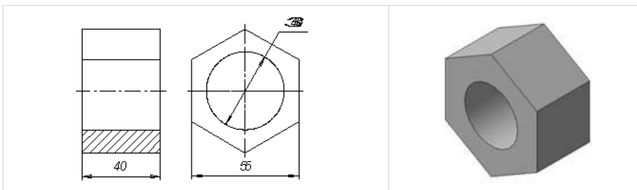
Рисунок 7.2 – Чертеж и модель гайки
