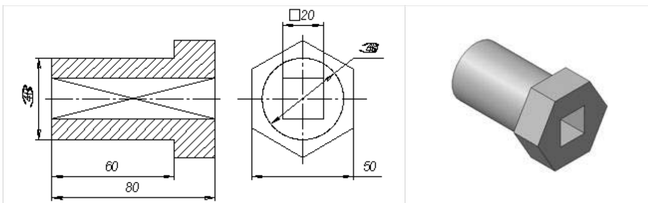
Рисунок 7.1 – Чертеж и модель вала
