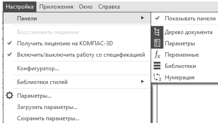
Рисунок 1.6 – Меню Настройка
