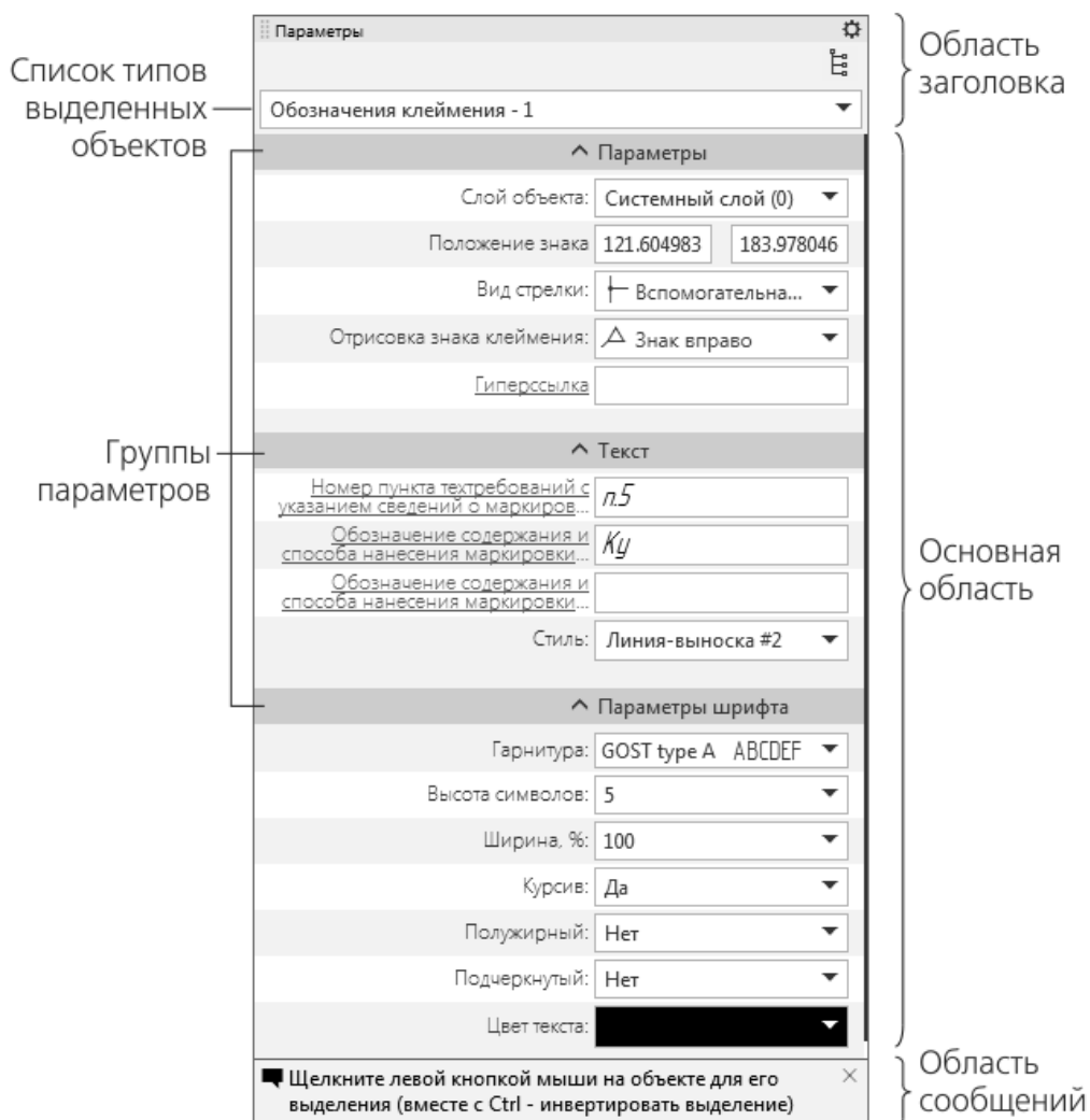
Рисунок 1.7 – Панель Параметры при изменении параметров объекта
