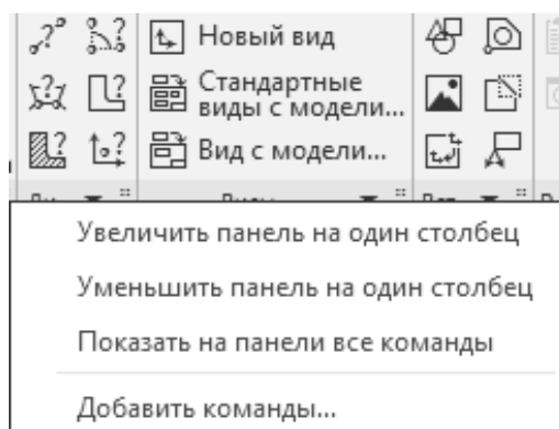
Рисунок 1.4 – Контекстное меню
