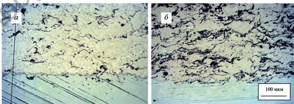
Рис. 6. Структура не травленных покрытий из порошков, полученных механическим легированием в течение 8 ч: а – ПН951О5; б – ПН851О15
