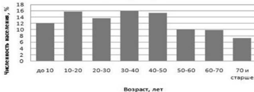
Рисунок 1.3 – Пример гистограммы
