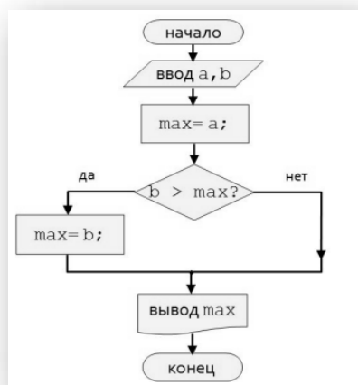
Рисунок 2.2 – Блок-схема неполного оператора if
