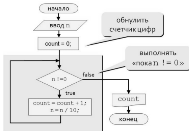
Рисунок 3.1 – Блок-схема подсчета количества цифр в числе
