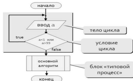
Рисунок 3.2 – Блок-схема организации ввода числовых данных
