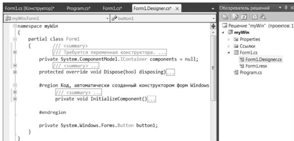
Рисунок 8.5 – Окно с автоматически создаваемым кодом класса Form1
