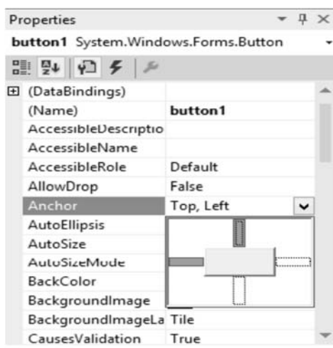
Рисунок 8.7 – Пример задания свойств Anchor (а) и Dock (б) для кнопки Button
