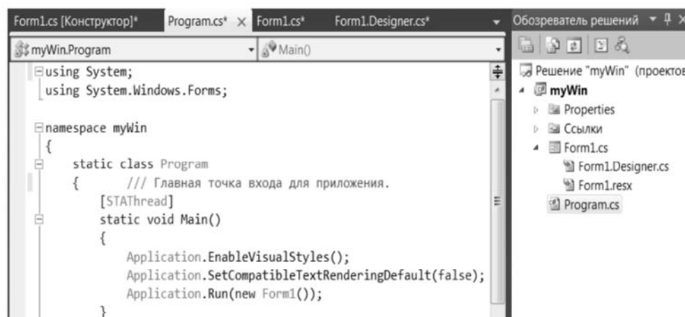
Рисунок 8.3 – Окно с кодом класса Program
