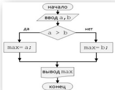
Рисунок 2.1 – Блок-схема поиска наибольшего из двух чисел
