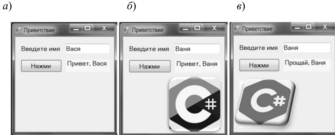
Рисунок 8.9 – Интерфейс приложения
