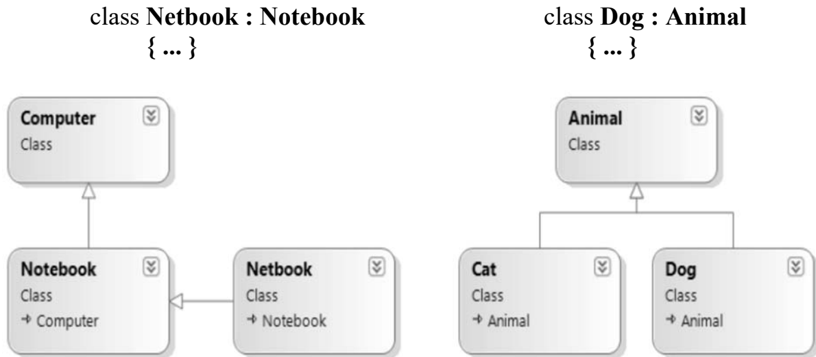
Рисунок 7.1 – Иерархии классов
