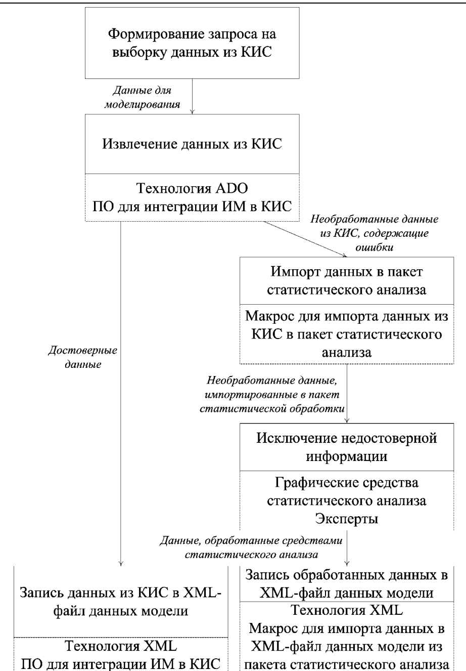
Рисунок 1 – Мониторинг ИС и получение данных для запитки ИМ
