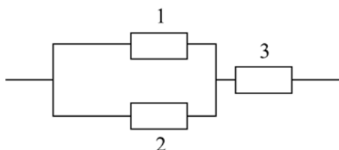
Рисунок 7.1 – Схема для расчета надежности
