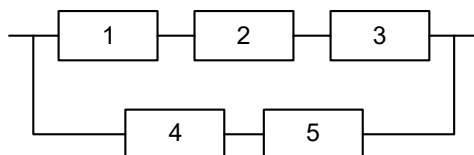
Рисунок 7.2 – Схема для расчета надежности
