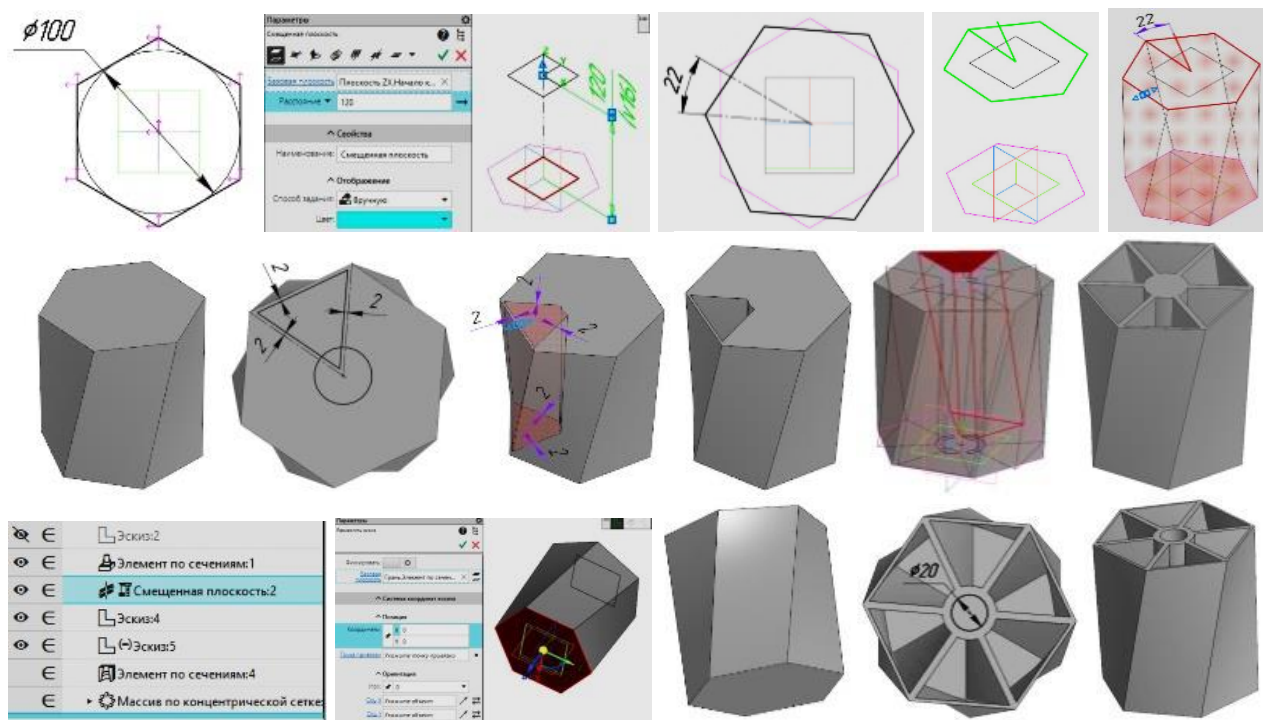
Рисунок 1 – Отдельные этапы выполнения модели в КОМПАС-3D
