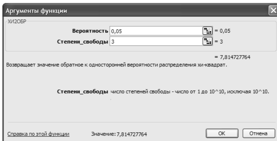
Рисунок 3.1 – Функция ХИ2ОБР
