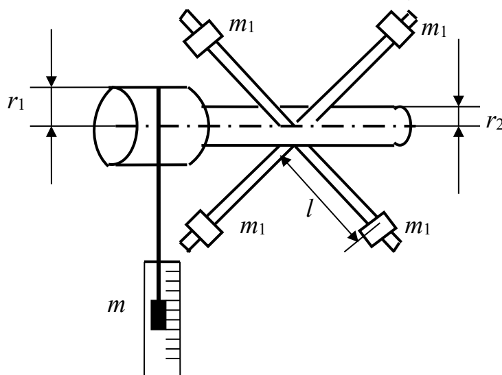
Рисунок 1.3 – Маятник Обербека
