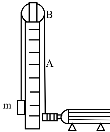
Рисунок 2.1 – Лабораторная установка
