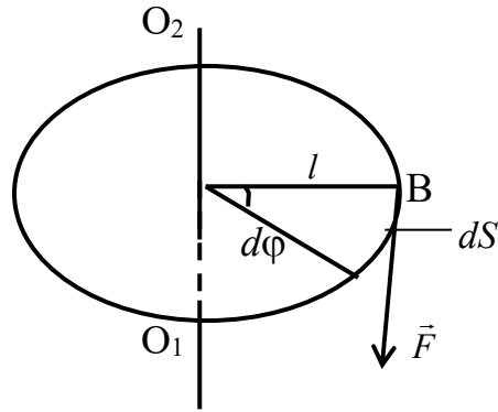
Рисунок 1.2 – Для вывода основного уравнения динамики вращательного движения
