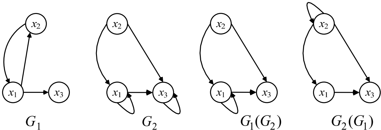
Рисунок 5 – Композиции графов
