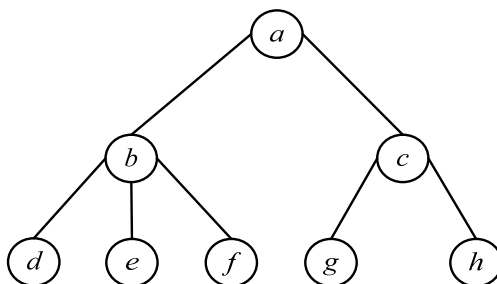
Рисунок 2 – Структура элементов множества
