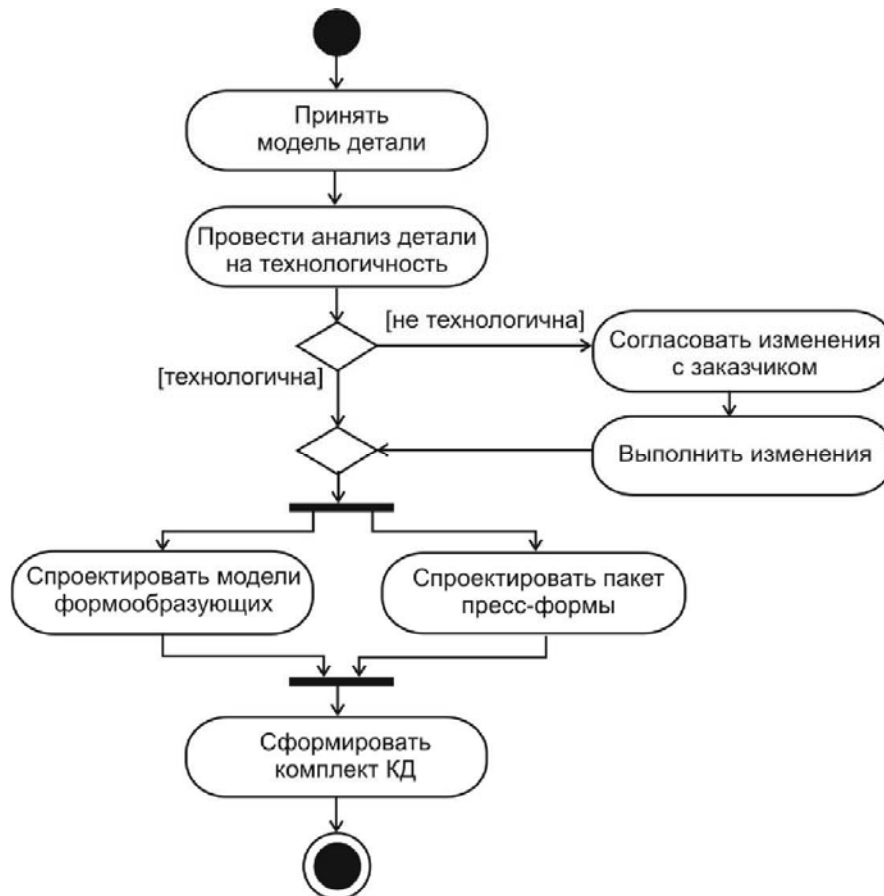
Рисунок 3 – Пример диаграммы деятельности
