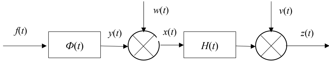
Рисунок 7.1 – Блок-схема объекта
