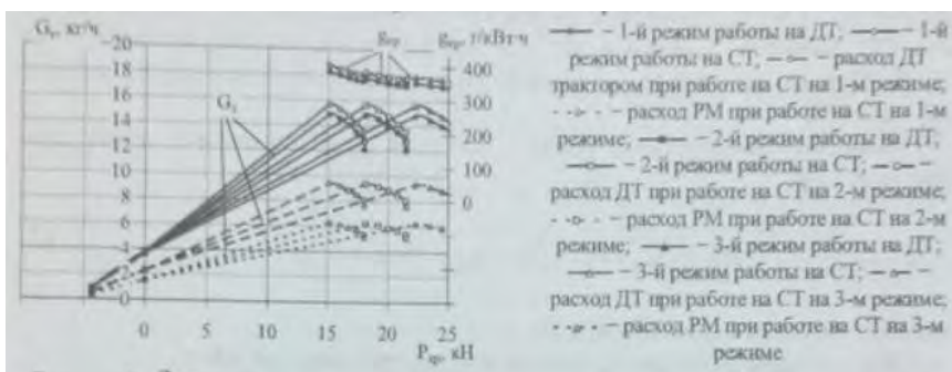
Рисунок 1 - Зависимость часовой и удельного расхода топлива трактора «БЕЛАРУС 922» от силы тяги на крюке при работе на ДТ м СТ, состоящем из 60 % ДТ и 40 % РМ
