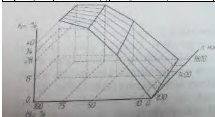
Рисунок 6 – Распределение состава смешеного топлива дизеля Д-245.5С2 в зависимости от частоты вращения и нагрузки при работе двигателя с системой регулирования
