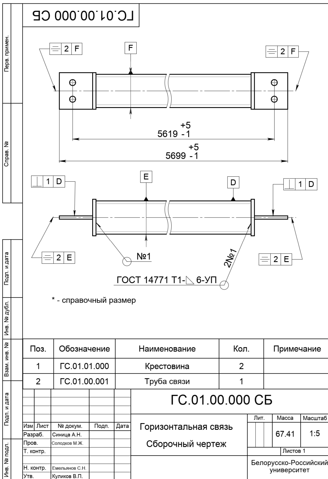
Рисунок 1.2 – Чертеж горизонтальной связи
