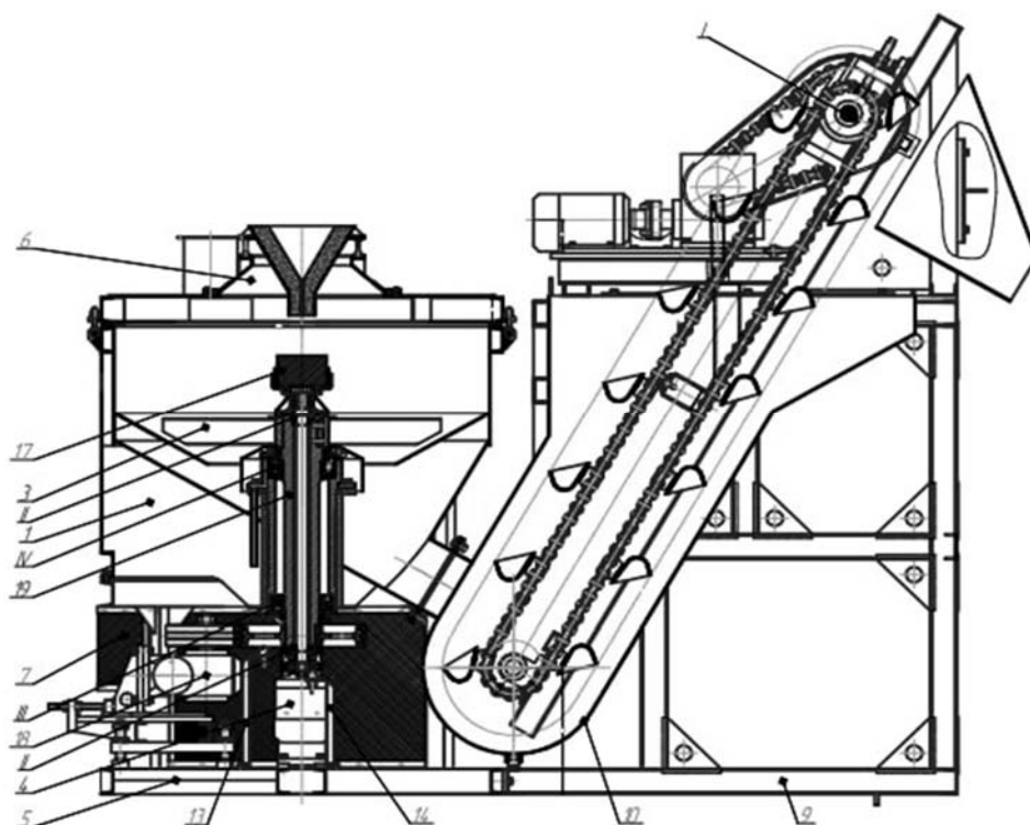
Рис. 1. Машина дробелитейная модели 46182М. Главный вид
