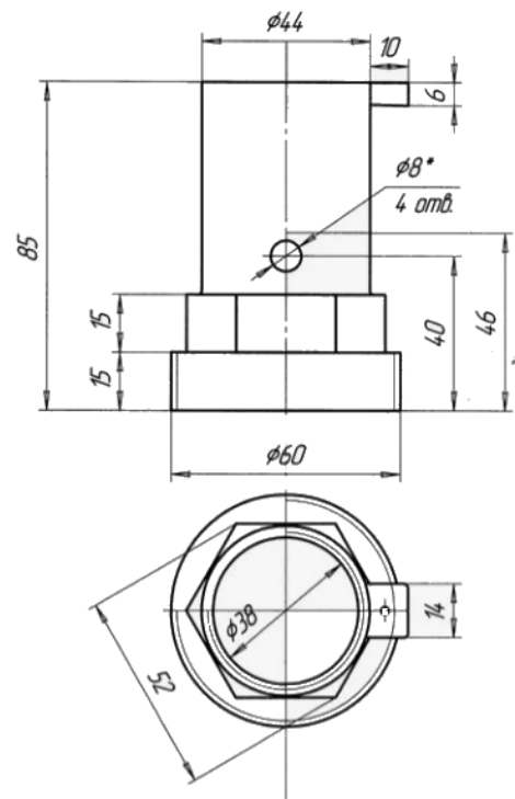
Рисунок 8.15 – Бугель
