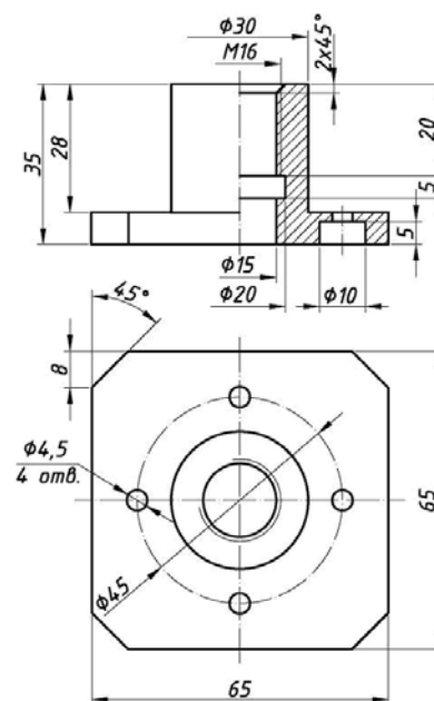
Рисунок 8.5 – Опора
