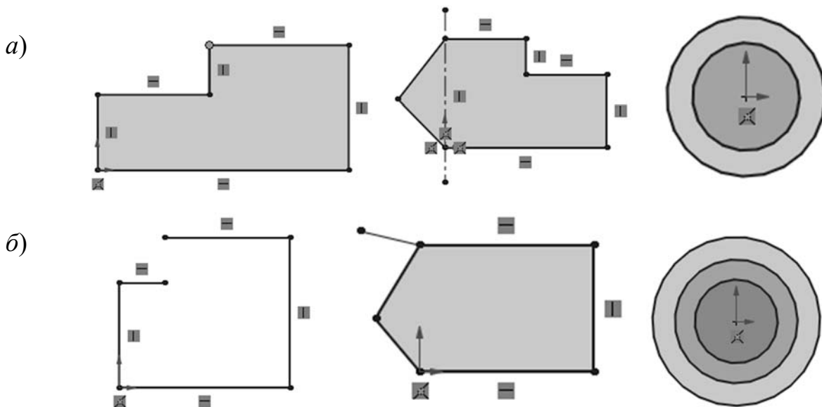
a – замкнутые эскизы; б – незамкнутые эскизы
