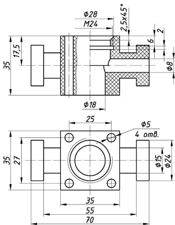
Рисунок 8.12 – Подушка
