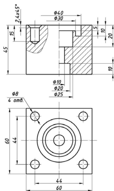
Рисунок 8.4 – Основание
