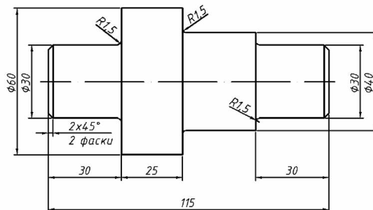
Рисунок 9.14 – Вал
