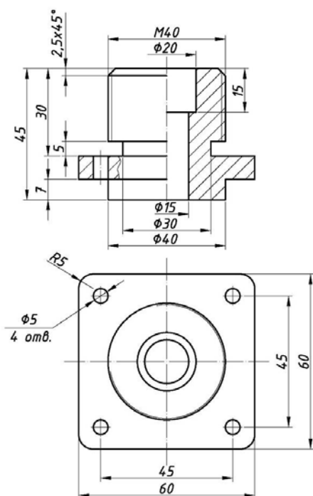
Рисунок 8.6 – Фитинг
