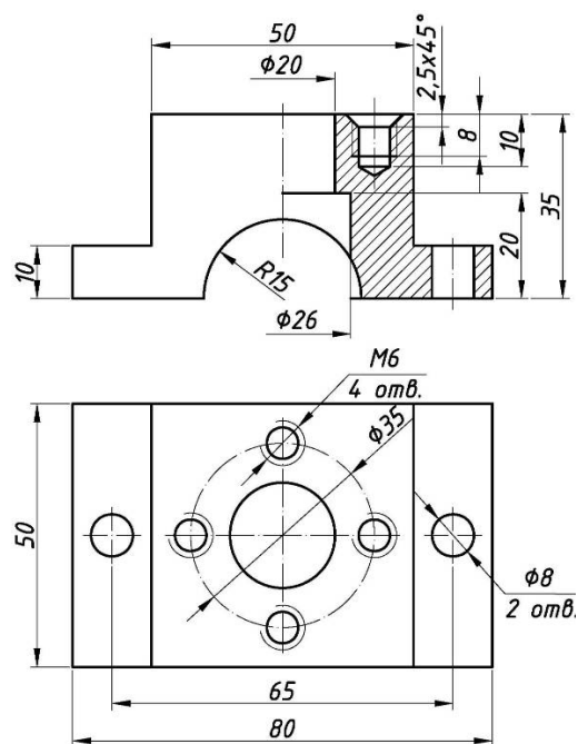
Рисунок 8.13 – Бугель
