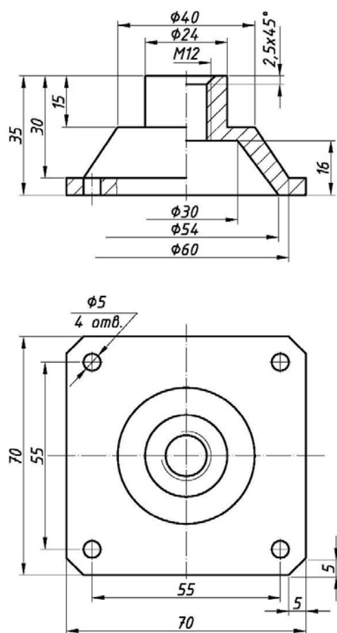
Рисунок 8.8 – Фланец
