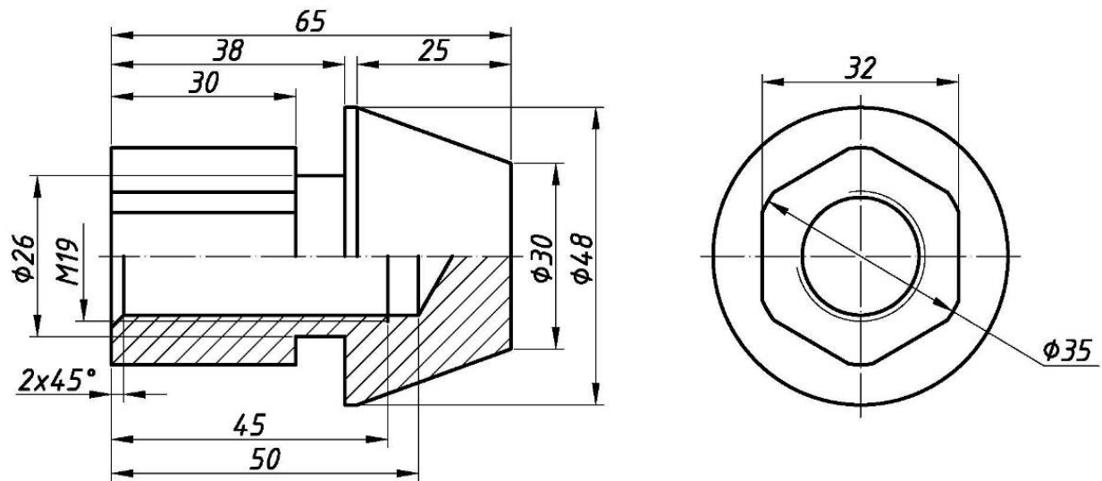
Рисунок 8.17 – Заглушка
