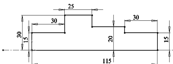
Рисунок 9.15 – Эскиз вала
