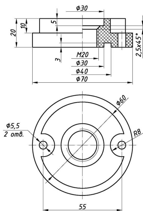
Рисунок 8.9 – Вставка
