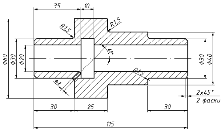
Рисунок 9.19 – Чертёж вала
