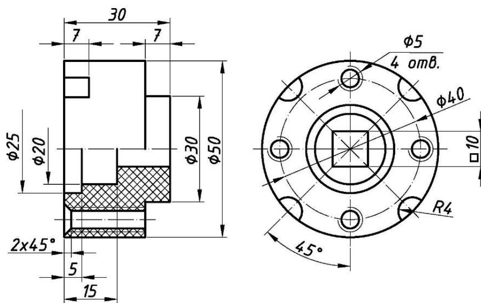
Рисунок 8.18 – Проставка
