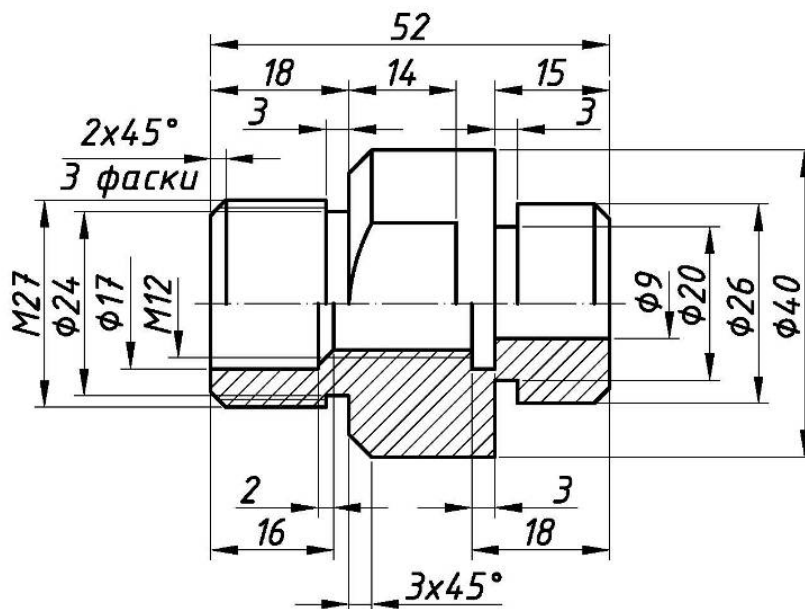
Рисунок 8.16 – Штуцер
