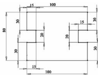
Рисунок 9.2 – Исходный эскиз
