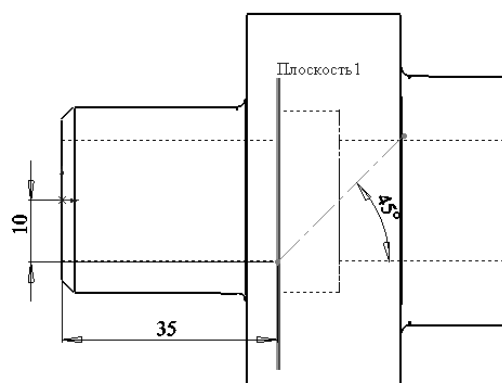
Рисунок 9.24 – Эскиз линии
