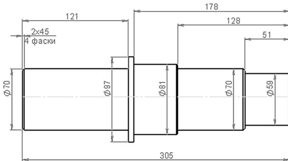
Рисунок 13.1 – Рабочий чертеж вала
