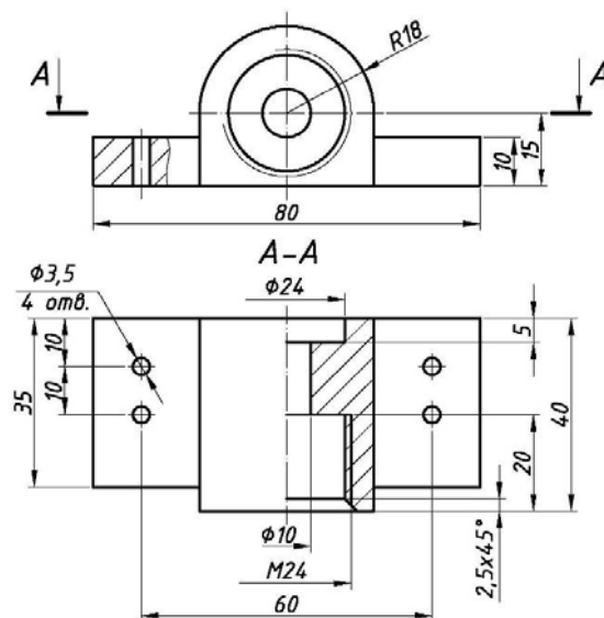
Рисунок 8.7 – Опора
