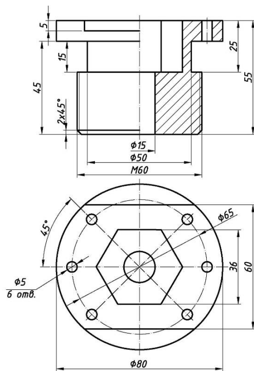
Рисунок 8.11 – Опора
