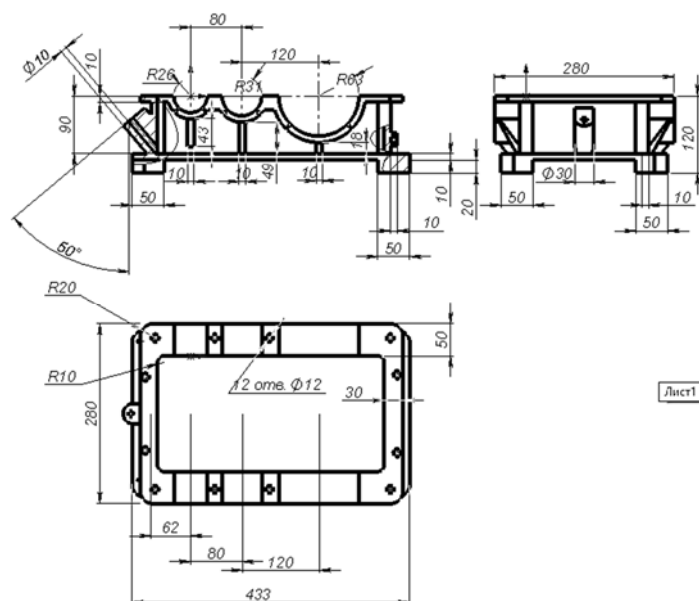
Рисунок 13.2 – Рабочий чертеж корпуса
