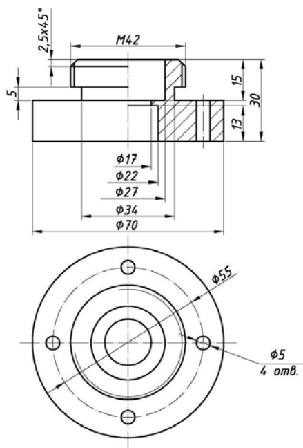
Рисунок 8.10 – Фланец
